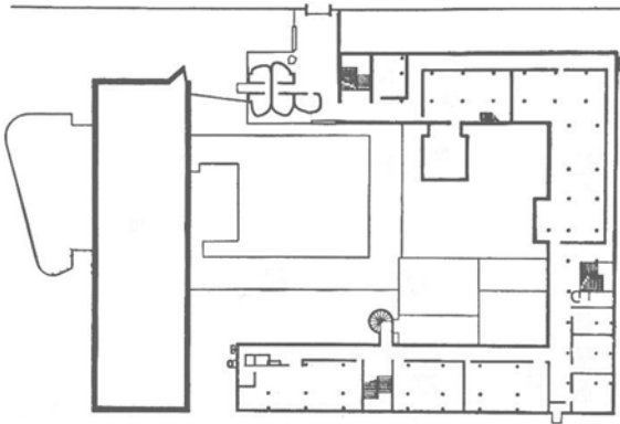
Zugangsgeschoss – Räume des Studiums und der Lehre. Planzeichnung Grundriss «Ebene 0»
