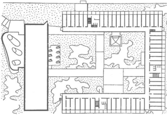
Obergeschoss – Räume des individuellen Rückzugs, Zellen der Brüder. Planzeichnung Grundriss «Ebene +1 und +2»
