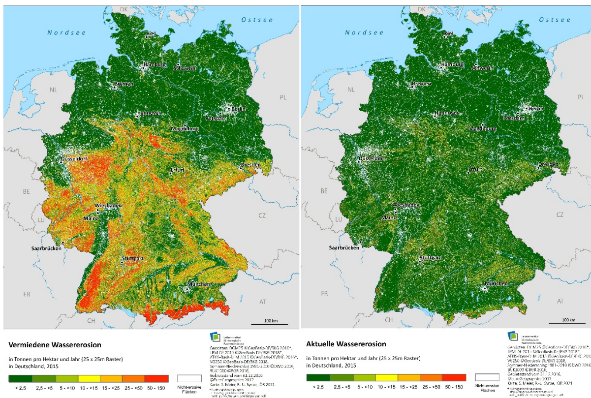
Abb. 4.4.1: Vermiedene Wassererosion 2015 (H), räumliche Auflösung: 25x25m.
