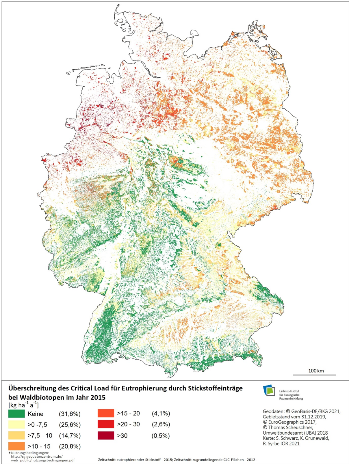
Abb. 3.7.5.2: Überschreitung des Critical Load für Eutrophierung durch Stickstoffeinträge bei Waldbiotopen im Jahr 2015
