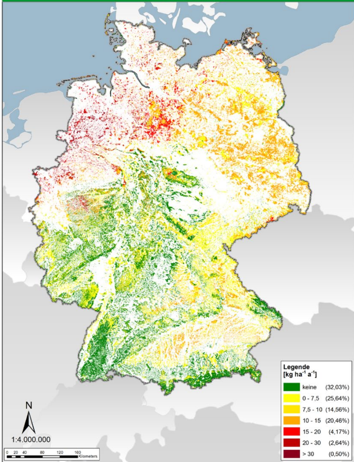
Abb. 3.7.5.1: Überschreitung der Critical Load für eutrophierenden Stickstoff im Jahr 2015. Quelle: UBA 2018 S.123
