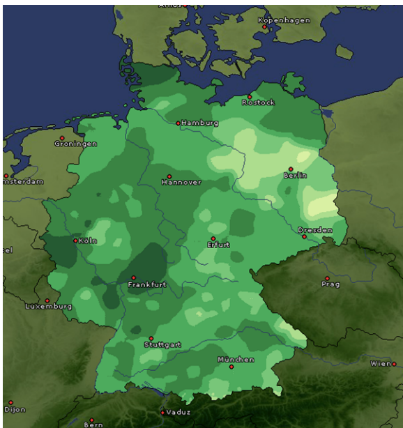
Abbildung 12: Erträge Winterweizen - 2,6^{\circ}\text{C} Erderwärmung
