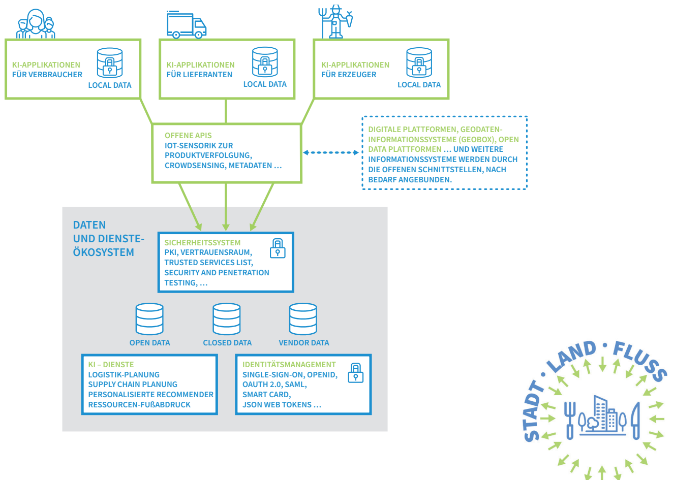
Abb. 2: Übersicht über die geplante KI-Plattformarchitektur im Verbundprojekt Stadt-Land-Fluss
