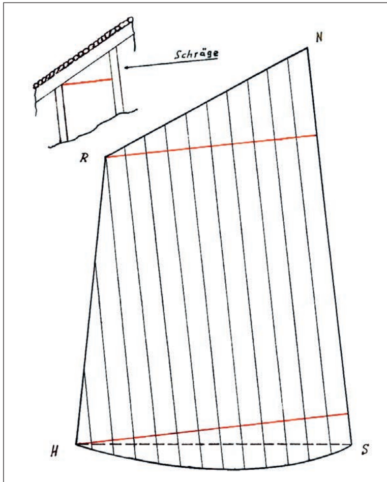
Abb. 33 Schnitt durch ein Schonse- gel nach Wil- helm Heincks: H = Hals; R = Rack; N = Nock (Gaffelnock); S = Schot. (Zeichnung: Verf.)
