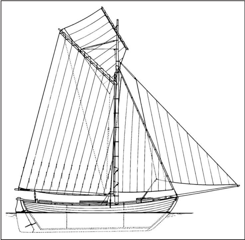
Abb. 18 Schwedisches Makrelenboot BLIXTEN, Besegelung mit Gaffelgroß, Fock, Klüver und Gaffeltoppsegel mit Rah. (Zeichnung: Staffan Claesson, Båtdokumentationsgruppen, Göteborg/Schweden)
