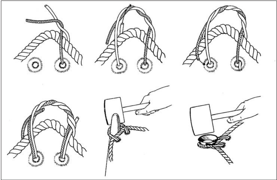
Abb. 47 Anfertigung eines Augspleißes an einer Nock. (Aus: Grohmann 1937)
