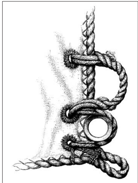
Abb. 50 Ausführung der Schotnock eines Bottersegels, gebändselt, Lägel mit und ohne Kausch. (Zeichnung: Peter Dorleijn)
