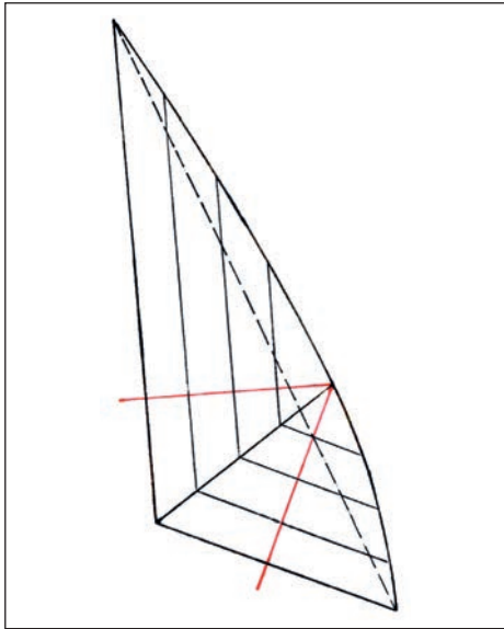
Abb. 32 Klüver mit Laschennaht nach Matthew Orr, nach Schaller. (Zeichnung: Verf.)
