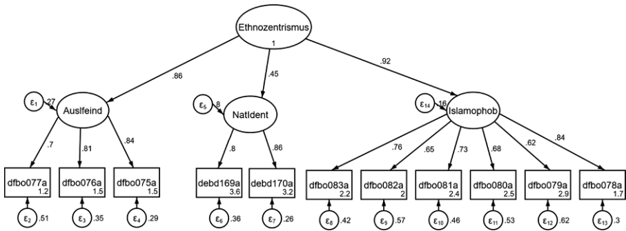
Abb. 1 CFA Ethnozentrismus. Quelle: GESIS (2018), eigene Berechnungen; Ausfeind Ausländerfeindlichkeit, Natldent nationale Identität, Islamophob Islamophobie
