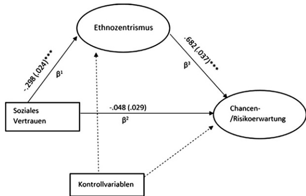
Abb. 5 Direkte und indirekte Effekte des sozialen Vertrauens und Erwartung von Flüchtlingszuwanderung. Quelle: GESIS (2018); eigene Berechnung; Full-Information-Maximum-Likelihood mit standardisierten Koeffizienten; Effektzerlegung soziales Vertrauen: indirekt \beta^3 * \beta^1 = -0,205 (0,023)***; total: \beta^2 + \beta^3 * \beta^1 = -0,253 (0,03)***; *** p < 0,001 , ** p < 0,01 , * p < 0,05 ; \beta^{1-3} (Koeffizienten aus der Berechnung zwischen den entsprechenden Variablen)
