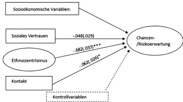
Abb. 6 Ergebnisse aus dem Modell 4. Quelle: GESIS (2018); eigene Berechnung; Full-Information-Maximum-Likelihood mit standardisierten Koeffizienten; *** p < 0,001 , ** p < 0,01 , * p < 0,05
