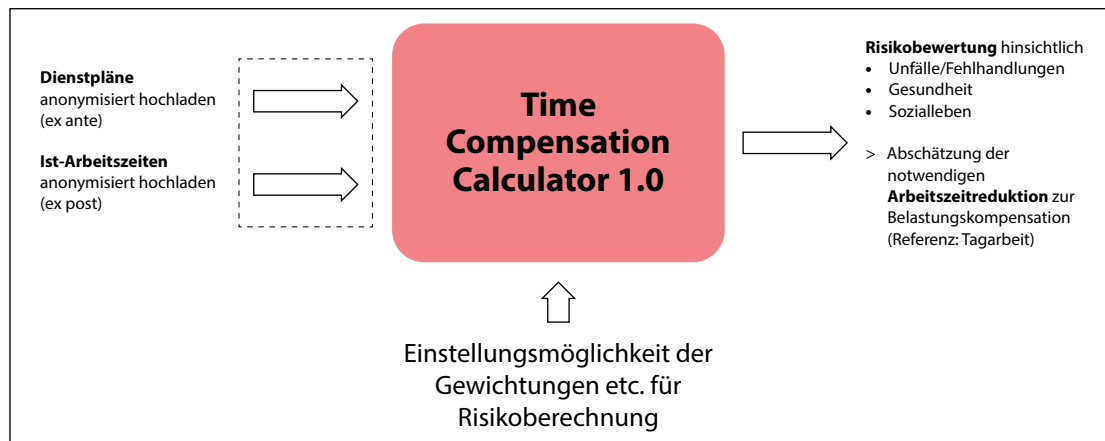
Abbildung 3: Schematische Darstellung des Time Compensation Calculator 1.0, einer Software-Lösung zur Risikobewertung von Arbeitszeitmodellen
