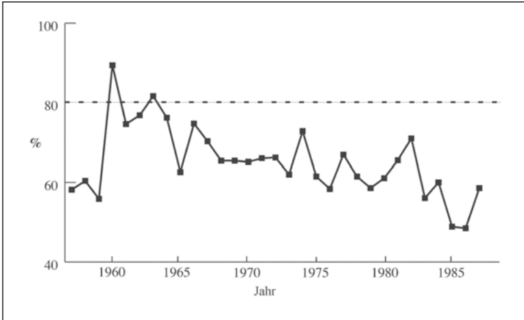
Abb. 4.2: Kalbungsrate
