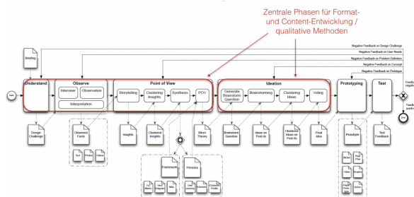
Abb. 3. Detailliertes Prozessmodell für Design Thinking
