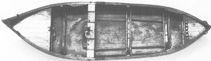
Das Modell während der ersten Restaurierungsphase. Der Fußboden ist entfernt und gibt die Fächerung zwischen den Knieen frei. Am Achterschiff sind die beiden Knaggen zu erkennen, deren Funktion noch unbekannt ist. (Foto: Egbert Laska, DSM)
