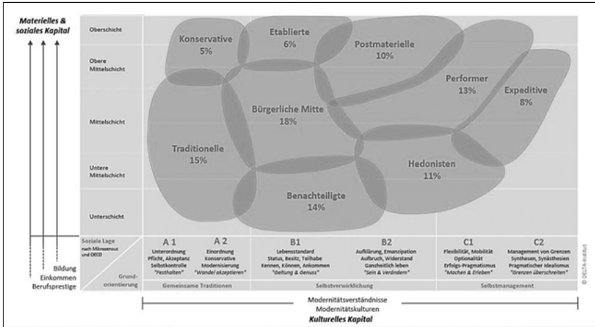
Abbildung 5: Die Delta-Milieus
