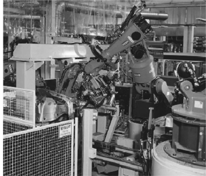
Abb. 2: Schweißroboter
