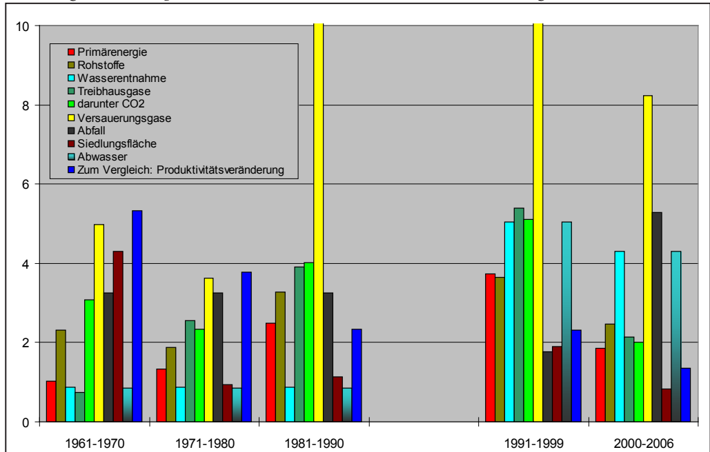
Abb. 2.3.-3: Durchschnittliche Veränderung der Ressourceneffizienz im Vergleich mit der Veränderung der Arbeitsproduktivität. Bis 1990 alte BRD, ab 1991 vereinigt Deutschland. **
