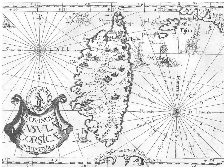
Abb. 17 Mittelländische Windrose
