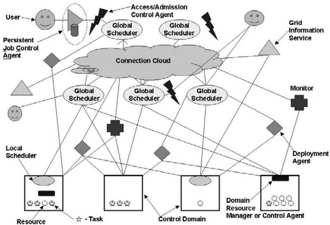
Hierarchisches Architekturmodell für das Grid-Resourcen-Management mit Cloud-Begriff für das Verbindungsnetz von 2000 64
