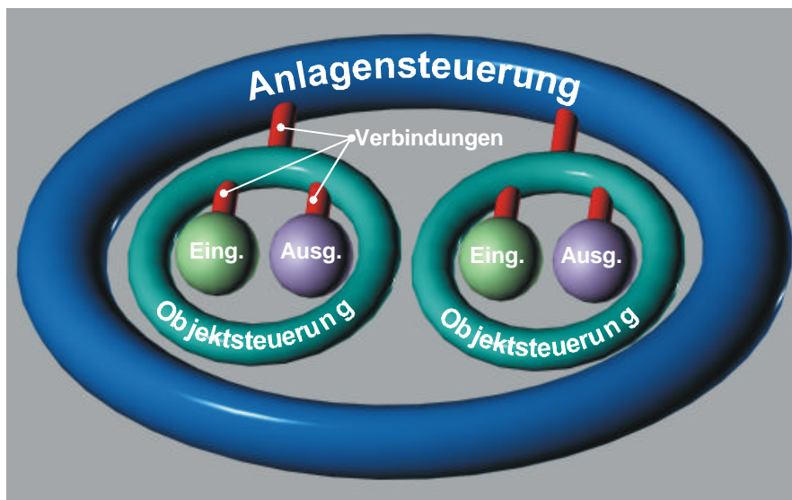
Abb 14: Hierarchisches Steuerungsmodell
