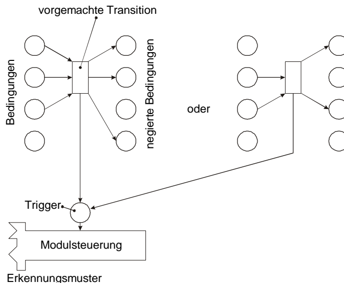
Abb 16: Vorgemachtes Steuerverhalten
