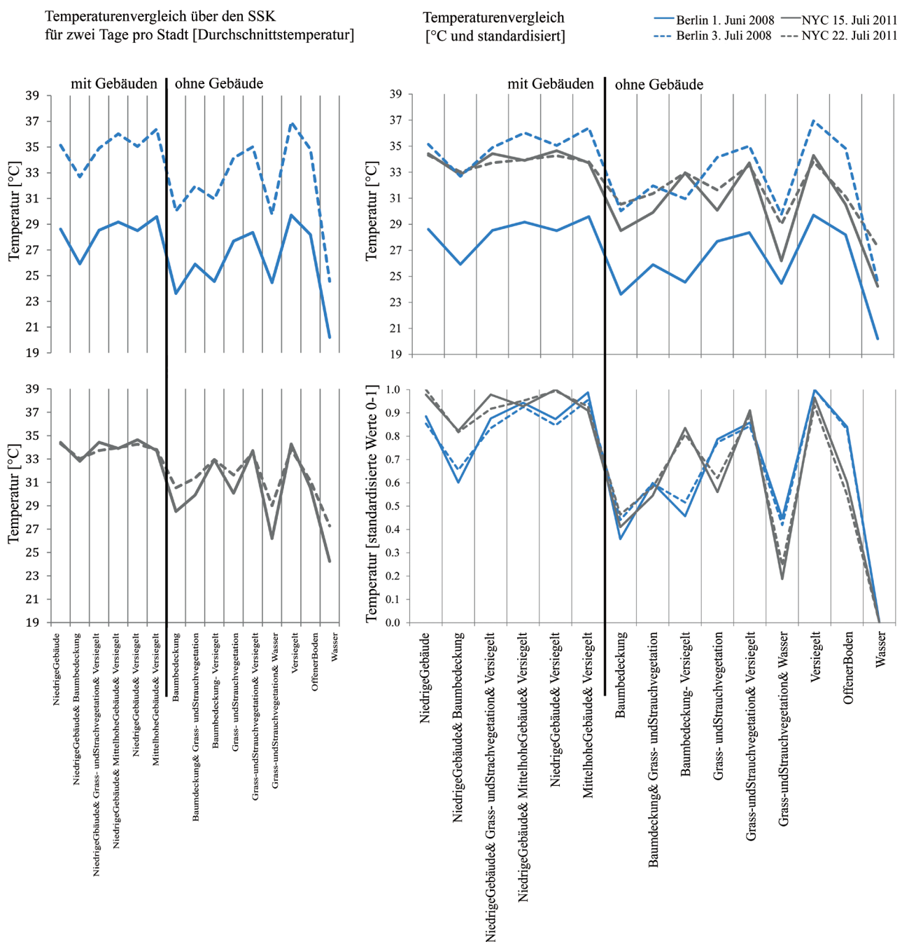
Abbildung 4: Temperaturverhalten über den gemeinsamen SSK (SSK geteilt in sechs bebaute Klassen (mit Gebäuden, links der schwarzen Linie) und neun unbebaute Klassen [rechts der schwarzen Linie]. Die linke Seite zeigt die Temperatur für zwei Tage in Berlin und NYC getrennt. Die rechte Seite zeigt die Temperaturen für beide Städte in einer Grafik [oben: Temperaturen für beide Städte; unten: Temperaturen für beide Städte; Min-Max-standardisiert])
