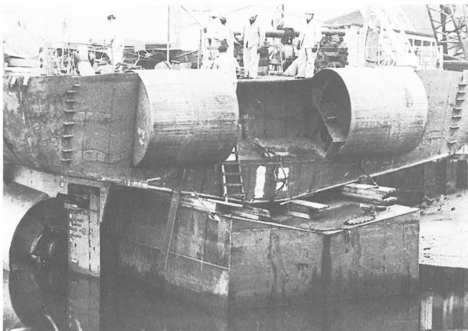
Abb. 21 Beim Stapellauf blieb der Bobrinzel Versorger BEN VIKING mit dem Heck im Krückau schlamm stecken und mußte mit Hilfe von Lufttanks wieder flottgemacht werden. Aufnahme 1975
