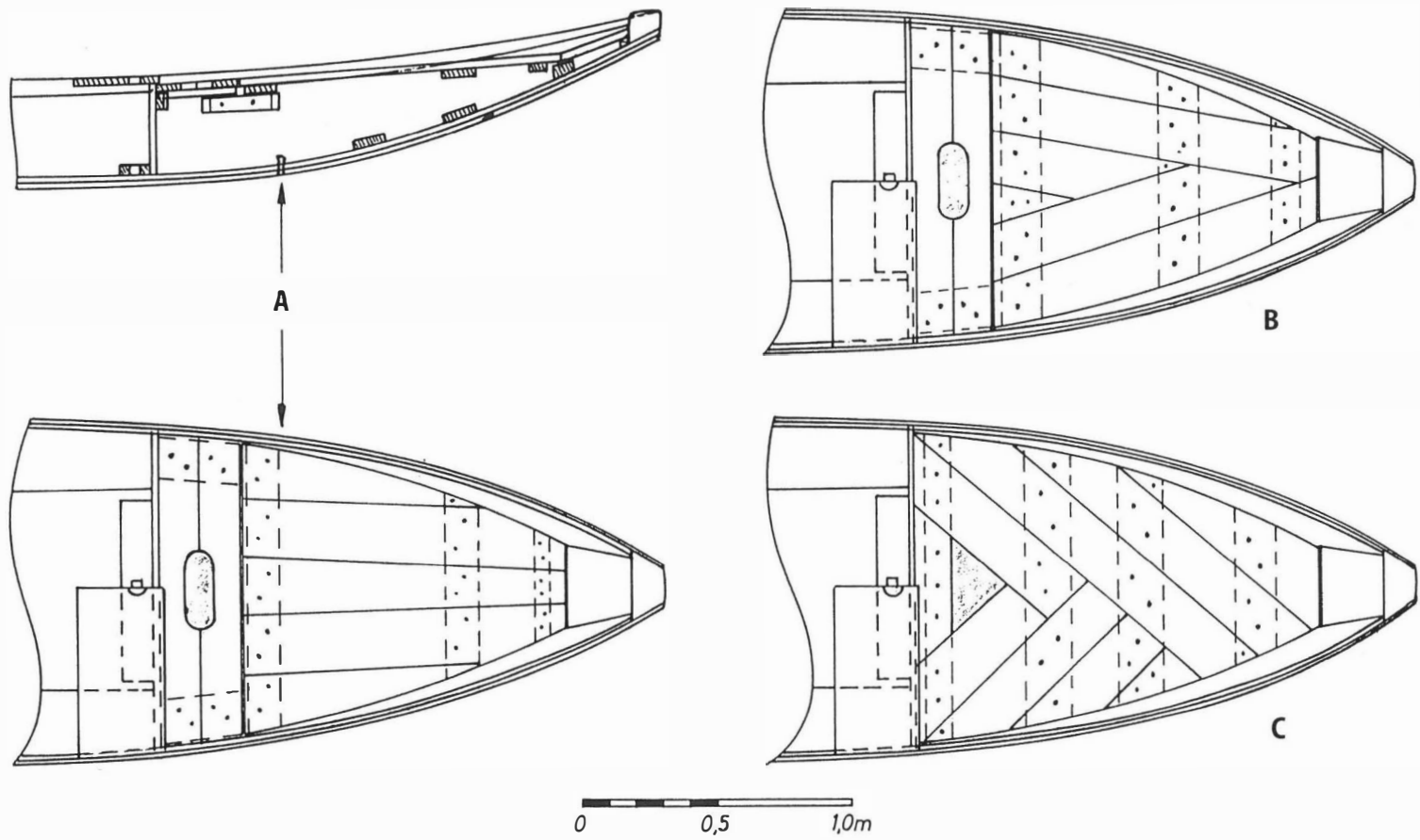
Die Schoor: Fischraum zur Kurzbälterung während des Fangs. A = allgemein übliche Ausführung; B, C = seltener vorkommende Varianten.
