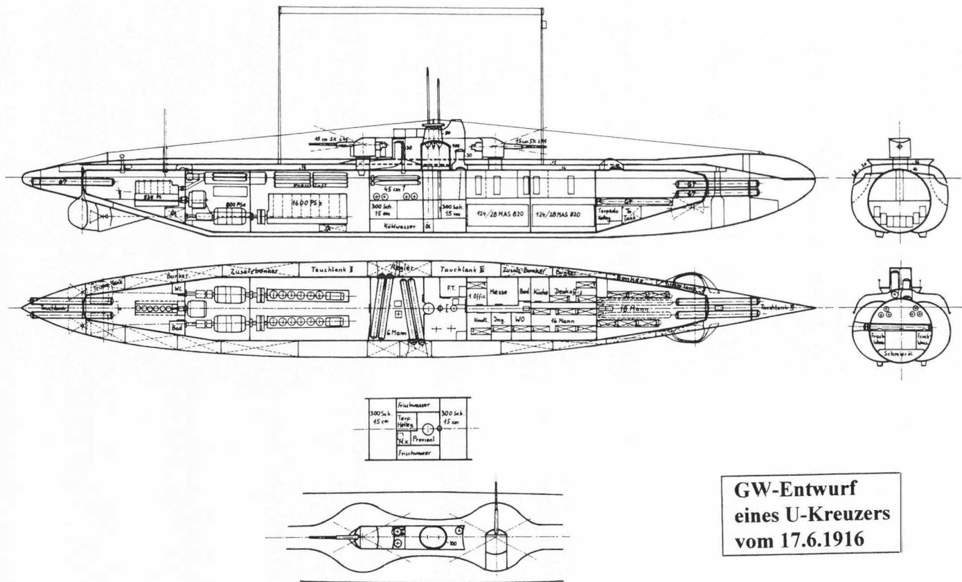
GW-Entwurf eines U-Kreuzers vom 17.6.1916.
