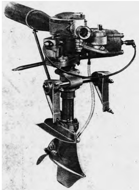
Rennbootmotor RM 175 DELPHIN aus Ludwigsfelde. (Archiv des Verf.)
