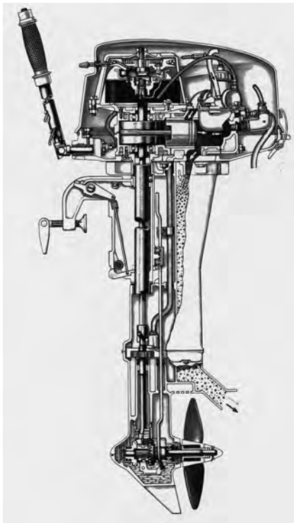
Schnittzeichnung der FORELLE (HB 125/1). (Archiv des Verf.)
