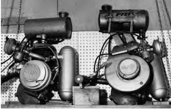
Der Magdeburger Außenborder PFEIL – ohne und mit Radialgebläse Kühlung. (Foto: Wolfgang Rudolph)
