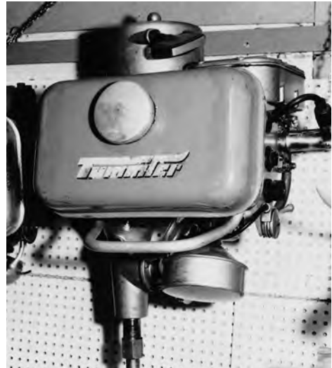
Außenbordmotor TUMMLER in jüngerer Ausführung. (Foto: Wolfgang Rudolph)
