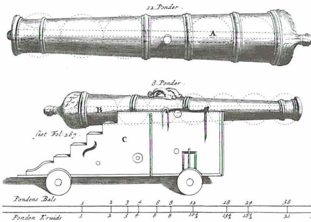
Abb. 6 12-Pfünder-Geschützrohr ohne, 8-Pfünder-Geschützrohr mit typischem Rapert, darunter Skala zum Verhältnis von Kugelgewicht zur Pulverladung; 1697
