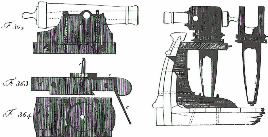
Abb. 10 Schiffsartilleristische Anschauungstafel mit Drehbassen damals modernster Art; 1798
