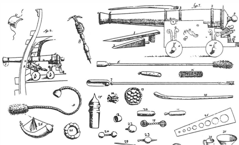
Abb. 5 Schiffartilleristische Anschauungstafel, 1691
