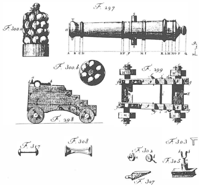
Abb. 7 Schiffsartilleristische Anschauungstafel, 1798
