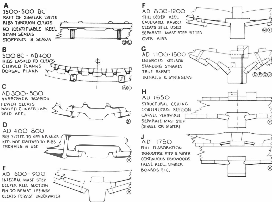
Abb. 4 Selbst Details von Schiffswracks können wertvolle Datierungshilfen in der maritimen Kulturlandschaft sein. Hier ein Versuch einer Übersicht über die Entwicklung des Kiels. (Eric McKee in: International Journal of Nautical Archaeology 1976, S. 4)
