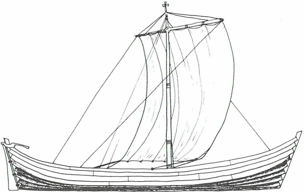
Abb. 22 Rekonstruktionszeichnung eines typischen Schiffes für die Innenfahrwasser, entwickelt auf der Grundlage des Fundes von Avafjärden, Löfvånger, Västerbotten, aus dem Ende des 15. Jhs. (Nach Seth Jansson: Båtfyndet från Avafjärden. C 1-Aufsatz in Archäologie an der Universität Umeå, 1981. Unpubliziert )
