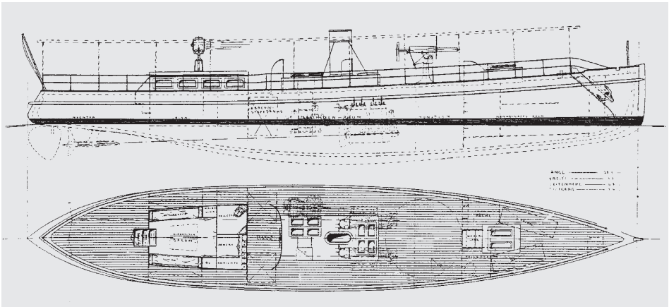
Abb. 12 Entwurf der Fr. Lürssen Werft in Aumund/Vegesack einer bewaffneten 21,90 m-Motoryacht, 1915. (Aus: Die Yacht 14/1915, S. 169)
