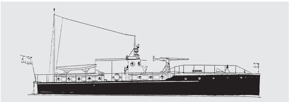
Abb. 14 Entwurf einer bewaffneten amerikanischen 19,80 m-Motoryacht von Lüders Marine Construction Co., 1916. (Aus: Die Yacht 37/1916, S. 458)
