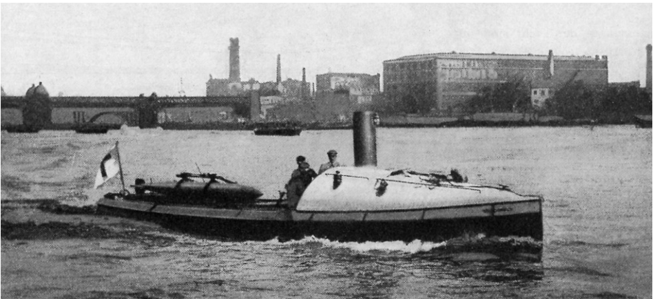
Abb. 13 Englische, mit einem Torpedo bewaffnete 56-Fuß-Motoryacht (100 PS) DRAGON FLY der Motor Boat Reserve (Royal Naval Volunteer Reserve), 1914. (Aus: Die Yacht 45/1914, S. 972)
