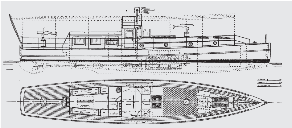
Abb. 1 Entwurf der Fr. Lürssen Werft in Aumund/Vegesack eines bewaffneten Motorbootes für die Türkei, um 1914. (Aus: Die Yacht 49/1914, S. 1017)
