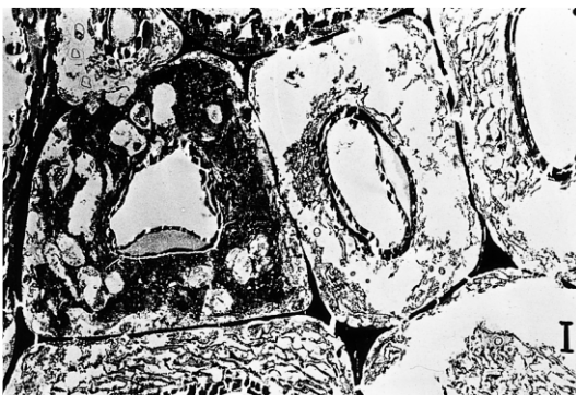
Abb. 13 Querschnitt durch stark abgebautes Ulmenholz: In der dunklen Zellwand der linken Zelle sind als rundliche Löcher die querschnittenen Kavernen von Moderfäulepilzen zu erkennen. Transmissions-elektronenmikroskopische Aufnahme bei etwa 3000facher Vergrößerung. (Aus: Hoffmann/Paramesvaran 1982)
