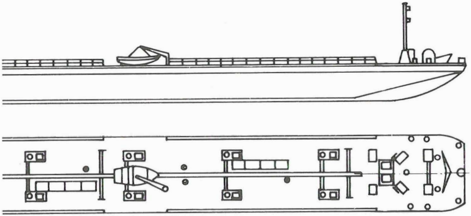
Bug eines Schubleichters (Tankleichters)
