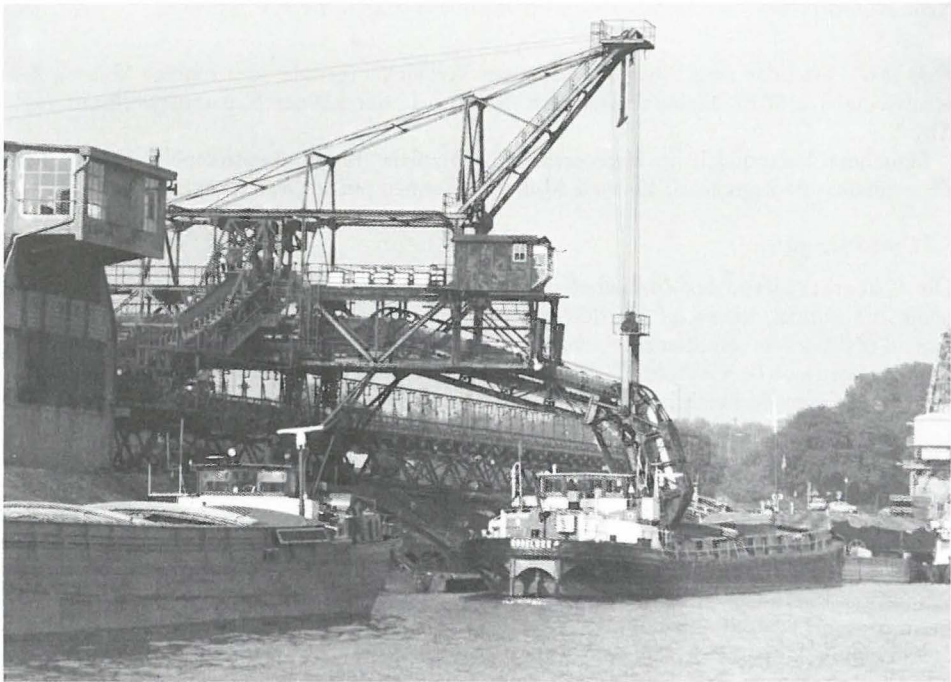
Alte Kohlenmischanlage im Ruhrorter Hafenbecken B (um 1980). Quer zum Bild das Zufuhrförderband. Der Laderüssel war in der Höhe und zur Breite hin verfahrbar. Die Anlage konnte am Kai entlangfahren und die Kähne beladen.
