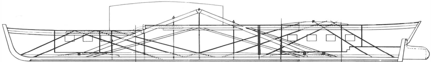
Plan der Verstärkung des Dampfers „Stadt Mainz“, Dezember 1833, nach Angaben von G. M. Roeslgen
