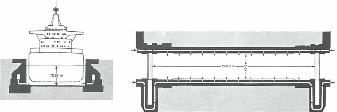
Abb. 10 Große Seeschleuse in Emden. (Nach: Seehafen Emden) Nach Inbetriebnahme des Dortmund-Ems-Kanals 1898 wurde ein neuer Massengutumschlaghafen geschaffen, der mittels einer Seeschleuse (1913) vom Gezeitenbereich der Ems abgeschlossen wurde. Zur damaligen Zeit ahnte man noch nicht, daß eines Tages 85 000-Tonner den Hafen anlaufen würden. Jahrzehntlang reichte die Kapazität der Schleuse völlig aus. Erst seit den sechziger Jahren zeigte sich, daß die Dimensionen der Seeschleuse den Anforderungen des Massengutseeverkehrs nicht mehr gewachsen waren.
