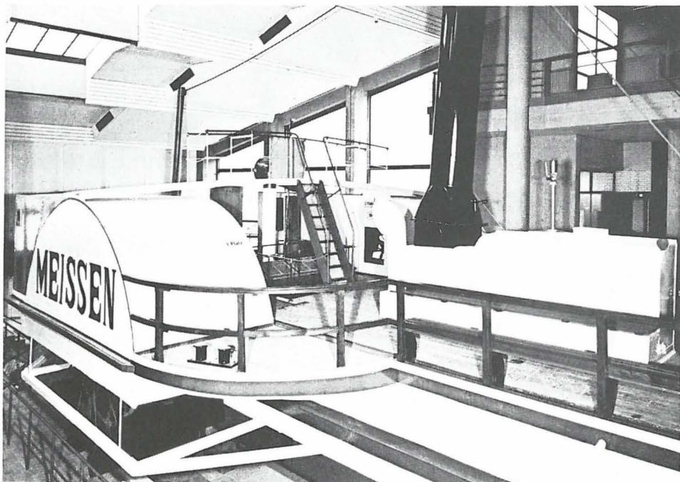
Abb. 18 Meissen fuhr von 1907 bis 1967 als Kronprinz Wilhelm auf der Oberweser. Das Mittelschiff befindet sich heute in seinem Ursprungszustand im DSM. (Foto: Meierdierks/DSM)
