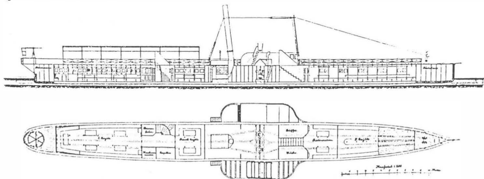
Abb. 21 Königstein, der Typ eines Schiffes um 1889. (Aus: Civilingenieur , 1890)
