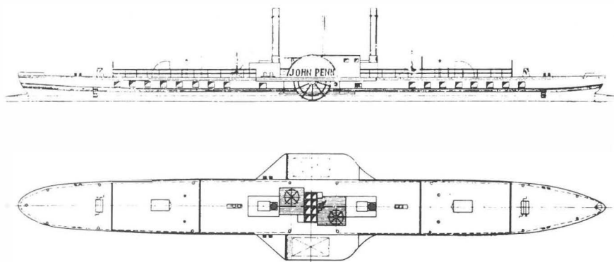
Abb. 10 John Penn als Schleppdampfer mit Personenbeförderung. Erstes Aussehen. (Rekonstruktionszeichnung J. Lüttich)
