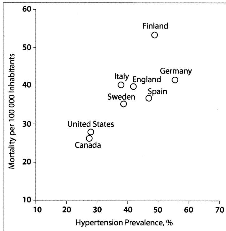
Abbildung 3: Zusammenhang zwischen der Prävalenz von Bluthochdruck und der Sterblichkeit in verschiedenen Europäischen und Nord-Amerikanischen Staaten (aus Wolf-Maier et al. 2003)
