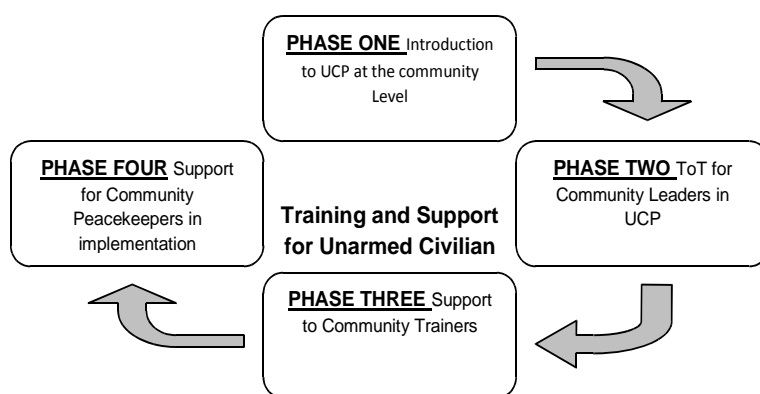
Bild 3 Trainingsphasen
