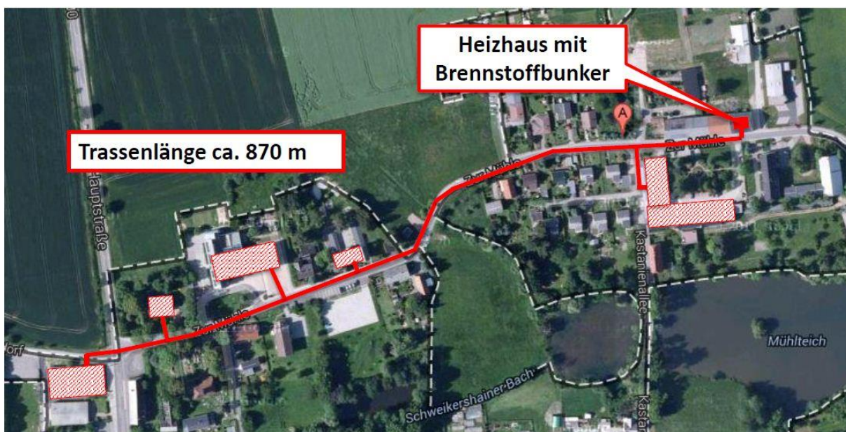
Abb. 13: Nahwärmenetz Schweikershain
