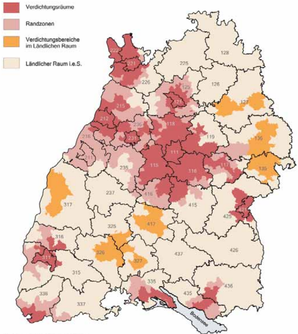
LEP 2002
