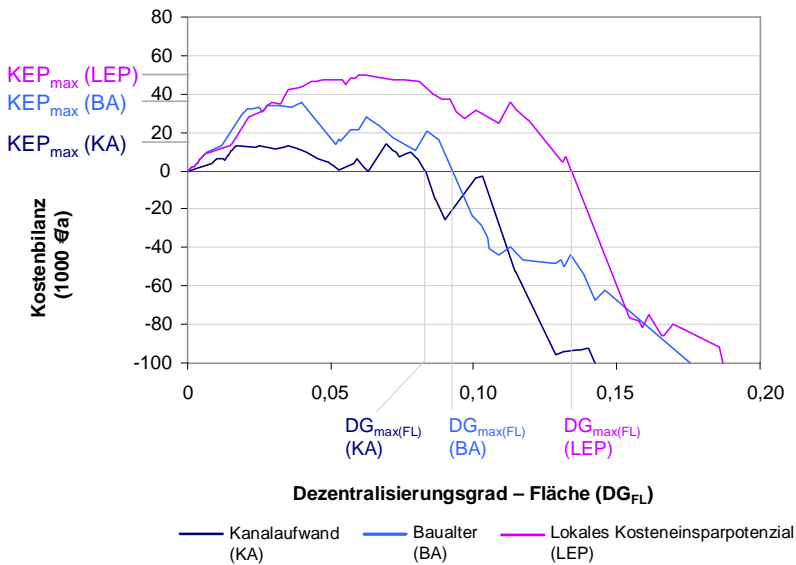
Abbildung 12-4: Kostenbilanzverlauf der Dezentralisierungspfade „Kanalaufland“, „Baualter“ und „Lokales Kosteneinsparpotenzial“ bezogen auf den Dezentralisierungsgrad (Fläche)
