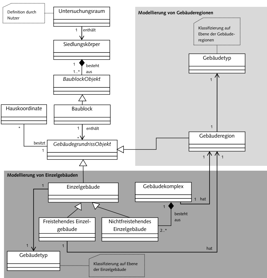
Abb. 5-3: Objekte des Siedlungsraums und deren Beziehungen im UML-Klassendiagramm
