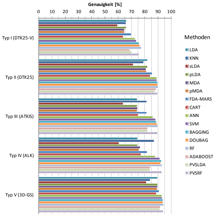
Abb. 8-10: Klassifikationsgenauigkeit der getesteten Klassifikatoren (Abkürzungen der Methoden entsprechend Kap. 7.8.2)
