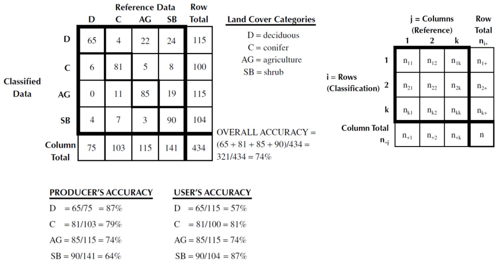
Abb. 3-11: Beispiel einer Konfusionsmatrix (links) und mathematischen Definition (rechts) (Quelle: Congalton & Green 1998)
