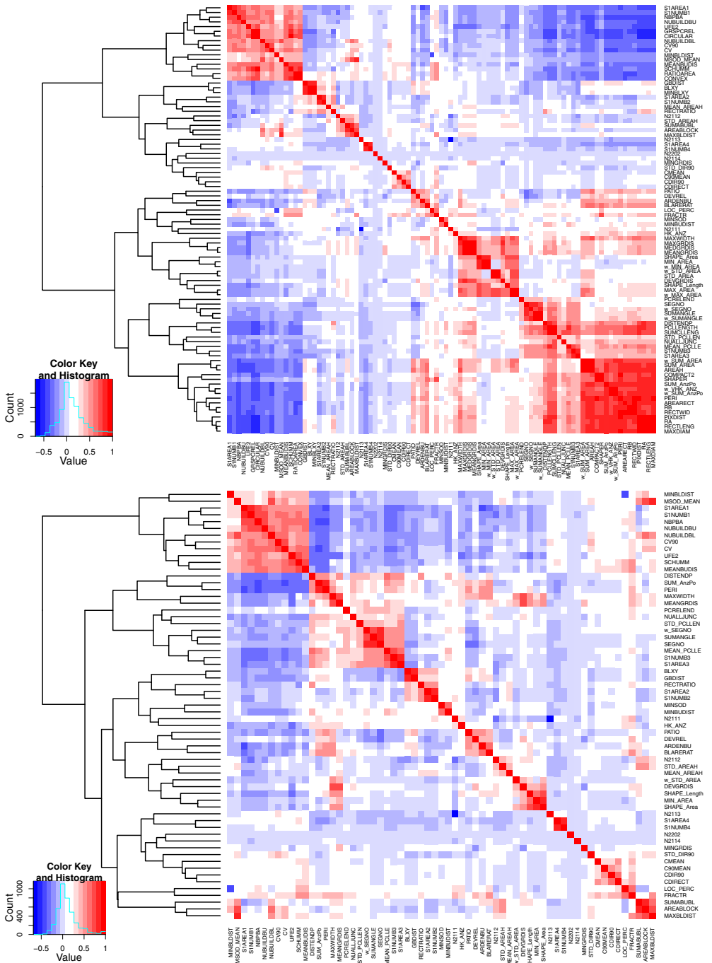
Abb. C-2: Visualisierte Korrelationsmatrix vor (oben) und nach (unten) der Merkmalsreduktion am Beispiel vom Datensatz Halle (Gebäude aus ATKIS® Basis-DLM)
