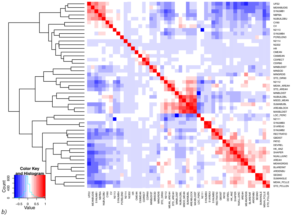
Abb. 8-9: Heatmap-Visualisierung der Korrelation der Merkmale vor (a) und nach der Merkmalsreduktion (b) am Beispiel der Daten von Halle – DTK25-V
