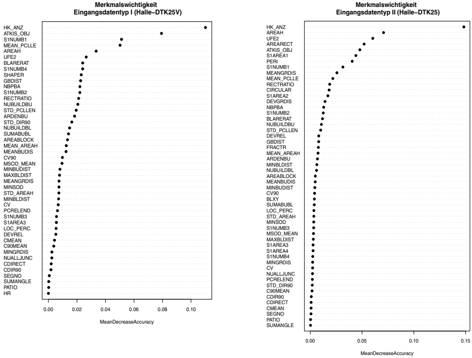
Abb. C-3: Merkmalswichtigkeit am Beispiel der Datensätze von Halle (DTK25-V und DTK25)
