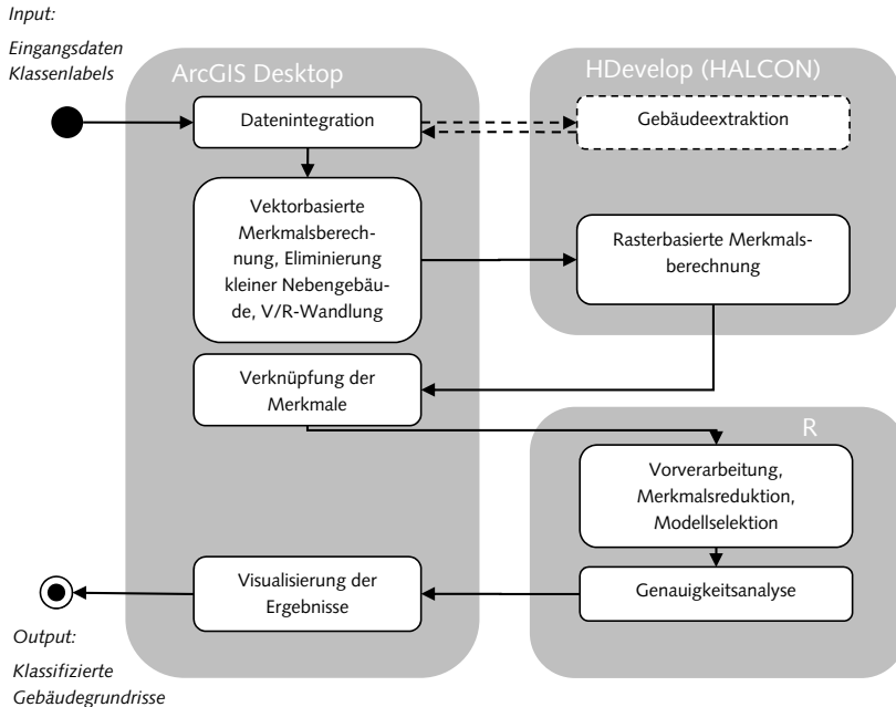
Abb. 7-15: Aktivitätsdiagramm der Verfahrensentwicklung
