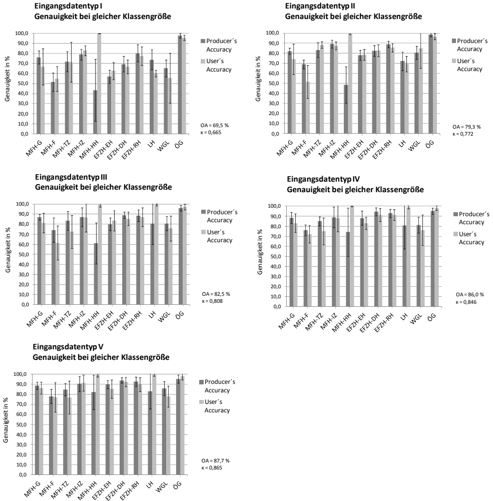
Abb. E-1: Klassenspezifische Genauigkeit verschiedener Eingangsdatentypen durch 10-fach wiederholtes Training und Testen anhand von 250 Trainings- und 250 Testobjekten pro Klasse (Fehlerbalcken gibt 2\sigma an).
