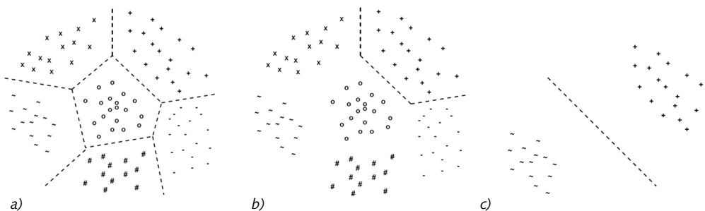
Abb. 3-9: Strategien zur Zerlegung des Mehrklassen-Problems (a) in binäre Teilprobleme nach OVO-Strategie (b) und der OVA-Strategie (c) (Quelle: Fürnkranz, 2001)
