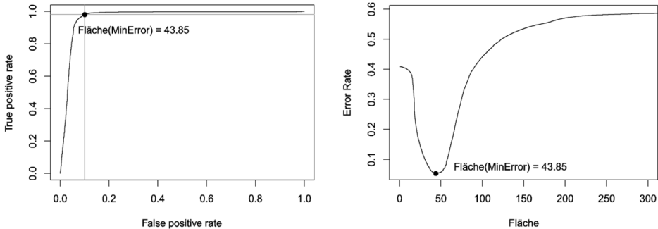
Abb. 7-11: Optimaler Schwellwert bei minimaler Fehlerrate am Beispiel kleiner freistehender Nebengebäude in der ROC-Kurve (links) und Fehlerkurve in Abhängigkeit der Messgröße Fläche (rechts)
