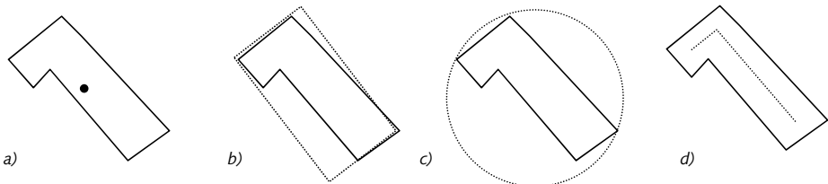
Abb. 7-9: Abgeleitete Hilfsobjekte: a) Flächenschwerpunkt, b) Kleinstes umschließendes Rechteck mit beliebiger Orientierung, c) minimaler Umkreis, d) Skeleton-Linie als Mittelachse der Gebäuderegion (Quelle: Eigene Darstellung)
