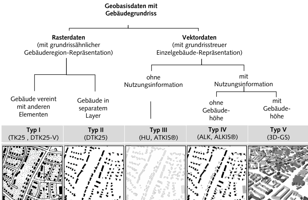
Abb. 7-4: Eingangsdatentypen
