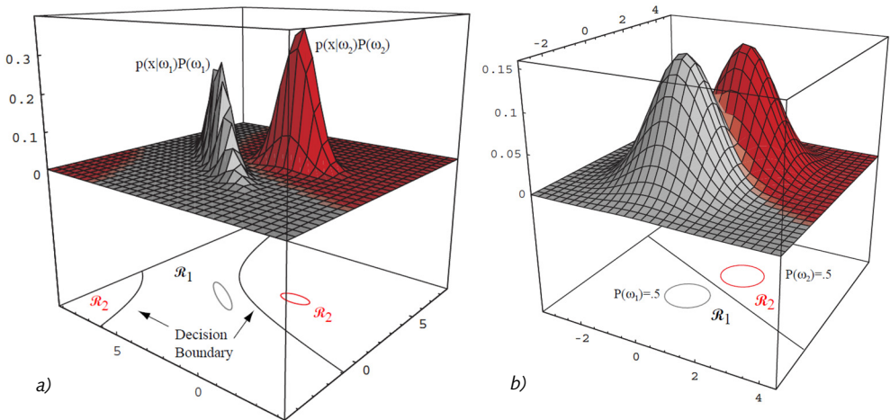
Abb. 3-6: 3D-Darstellung zweidimensionaler Verteilungsdichten und optimale Trennung nach dem Bayes-Theorem: a) normalverteilte Verteilungsdichten zweier Klassen mit unterschiedlichen Kovarianzmatrizen (optimale Trennung entspricht quadratischer Trennfunktion) b) normalverteilte Verteilungsdichten zweier Klassen mit identischen Kovarianzmatrizen (optimale Trennung durch lineare Trennfunktion) (Quelle: Duda et al., 2000)
