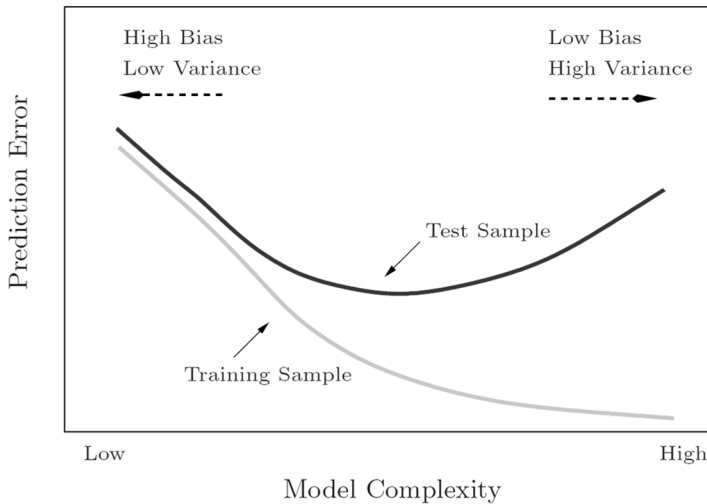
Abb. 3-10: Zusammenhang zwischen Vorhersagefehler und Modellkomplexität (Quelle: Hastie et al., 2009)
