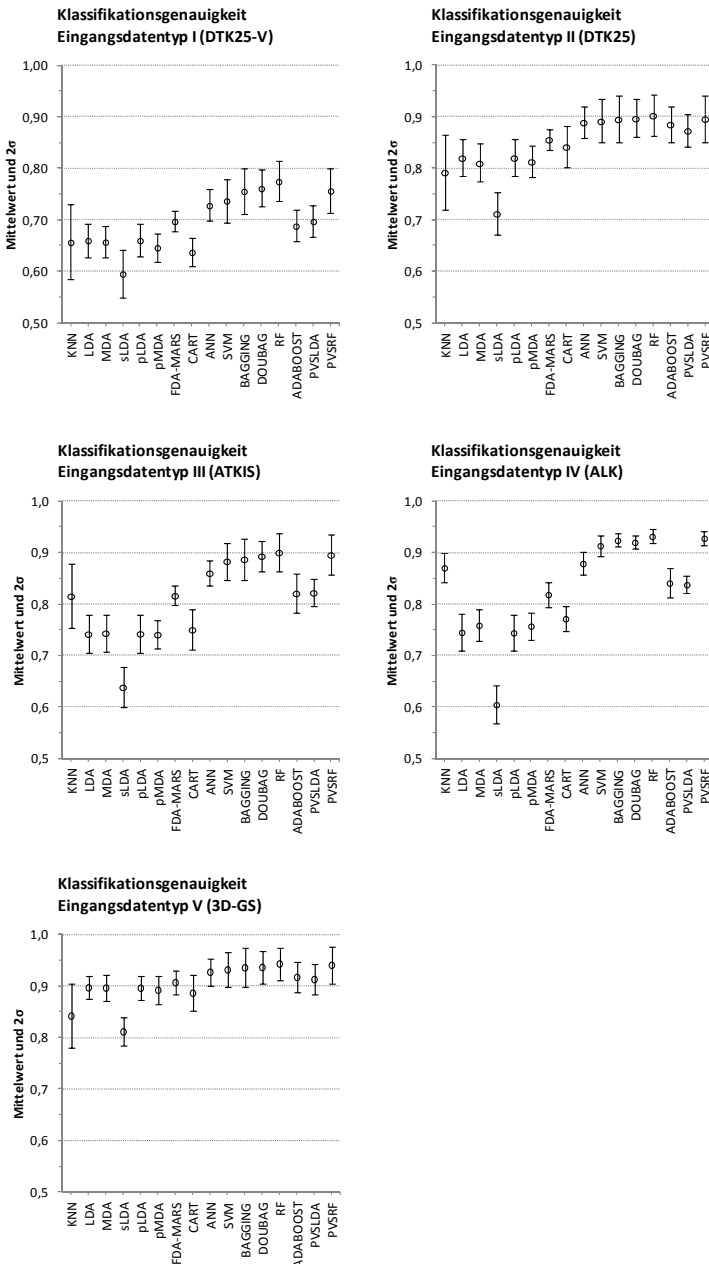
Abb. D-3: 10-fach kreuzvalidierte Klassifikationsgenauigkeit der getesteten Klassifikationsverfahren und deren Streuung (zweifache Standardabweichung 2\sigma ) anhand verschiedener Eingangstypen bei einer Lerndatenmenge n = 10\,000
