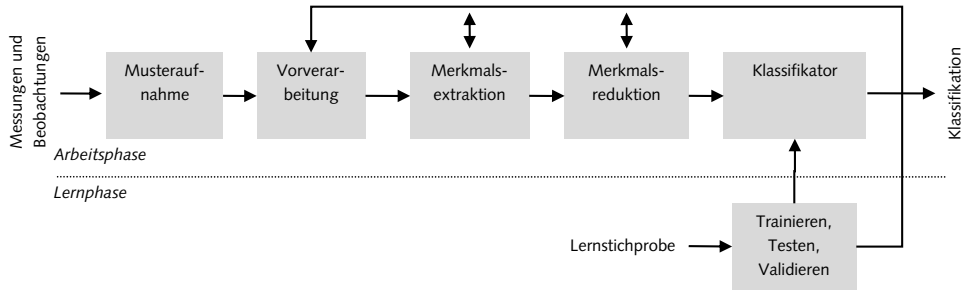
Abb. 3-3: Schema eines Mustererkennungssystems (Quelle: Eigene Darstellung in Anlehnung an Niemann 2003; Theodoridis & Koutroumbas 2008; Schalkoff 2008)
