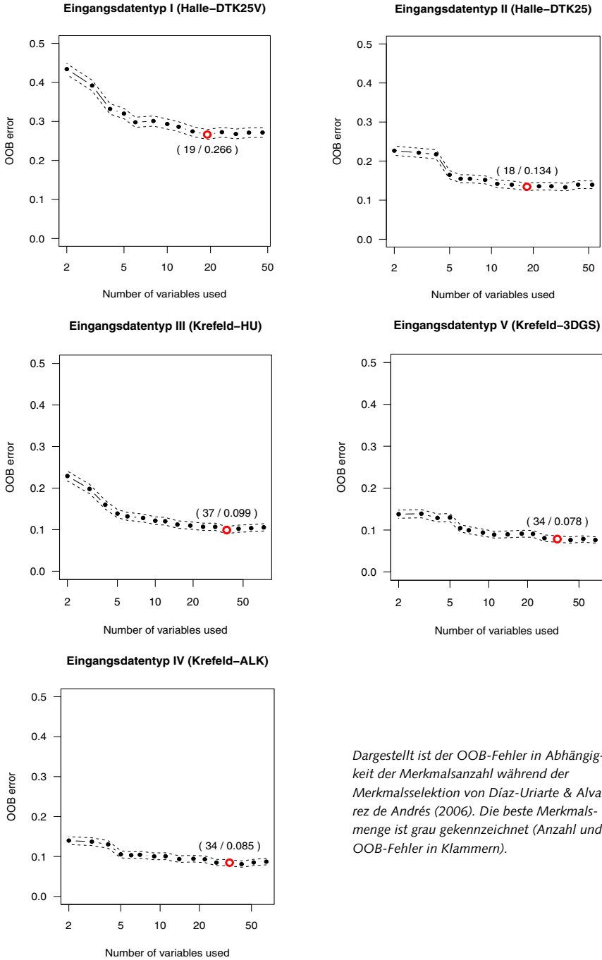
Abb. C-6: Ergebnisse der Merkmalsselektion mittels Random Forest
