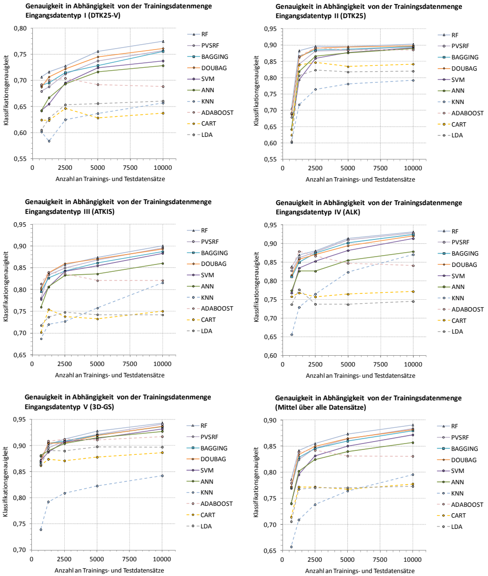
Abb. 8-11: Klassifikationsgenauigkeit in Abhängigkeit des Umfanges der Trainingsdatenmenge
