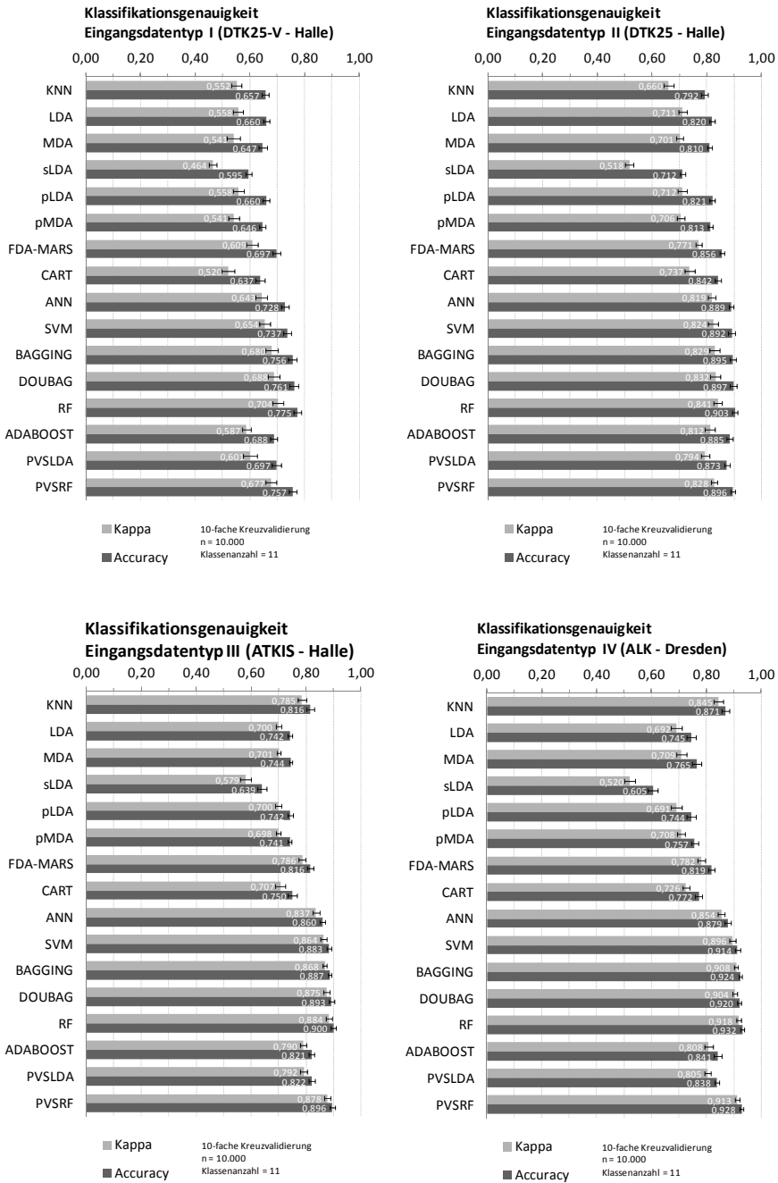
Abb. D-1: Klassifikationsgenauigkeit (Overall Accuracy und Kappa) für die Eingangstypen I-IV
