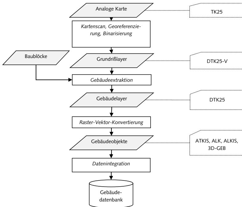
Abb. 7-5: Semantische und geometrische Harmonisierung der verschiedenen Datenmodelle
