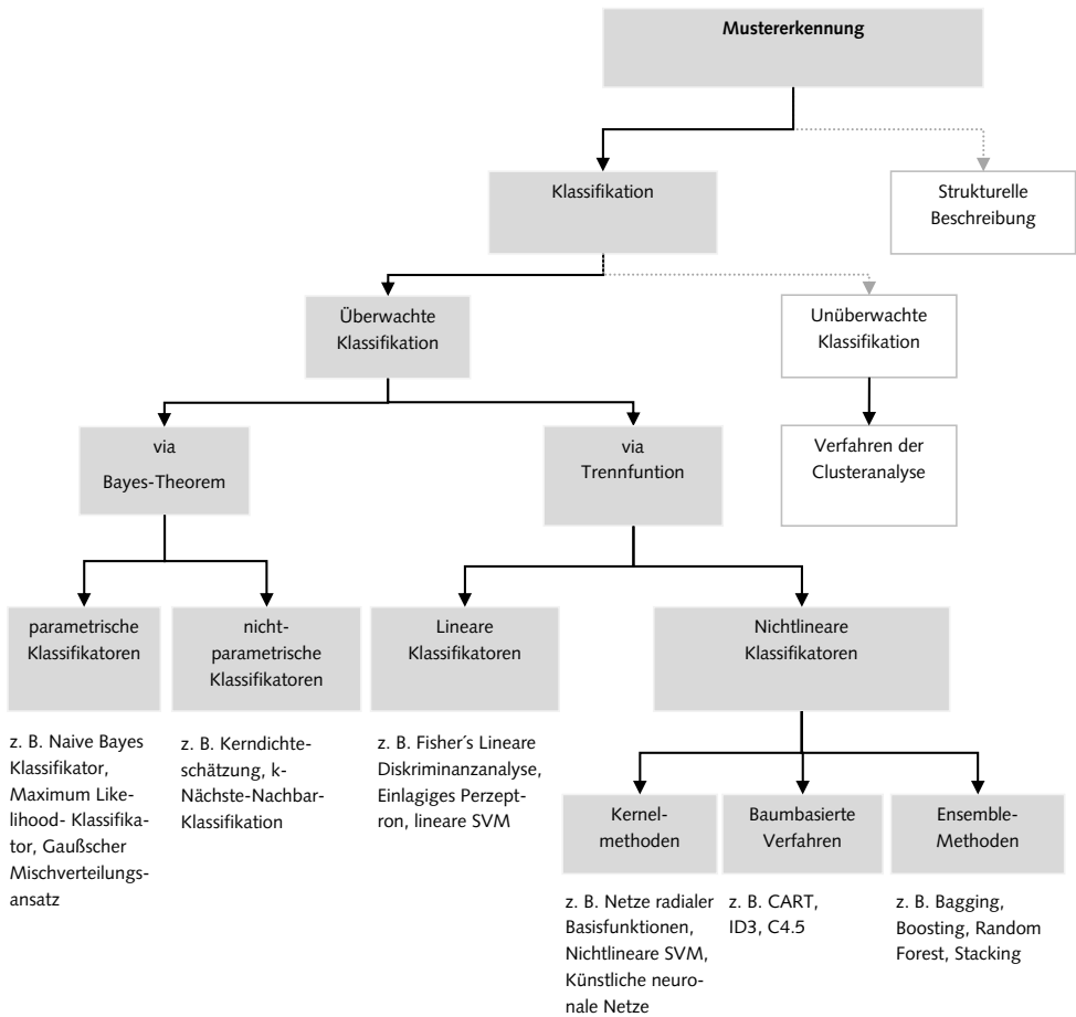
Abb. 3-4: Klassifikationsverfahren (angelehnt an A. R. Webb 2002)
