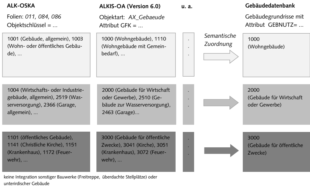
Abb. 7-6: Semantische Transformation der Nutzungsklassen in die drei verfahrensspezifischen Klassen am Beispiel der ALK und dem ALKIS (Eingangsdatentyp IV)
