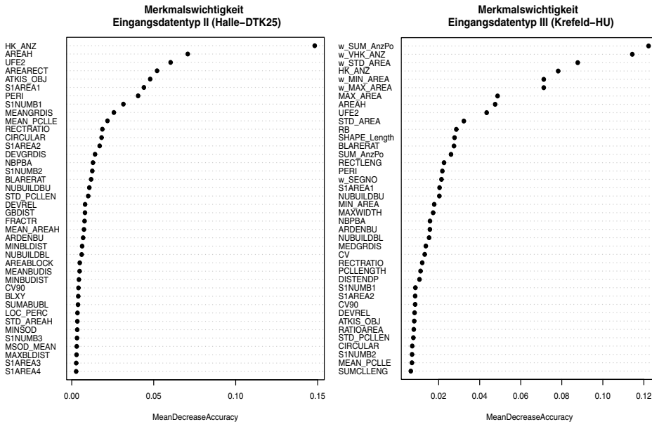
Abb. 8-19: Merkmalschwichtigkeit (PIM) gemessen am mittleren Genauigkeitsverlust (Mean Decrease Accuracy) beim Weglassen des Merkmals am Beispiel der Eingangsdatentypen II und III
