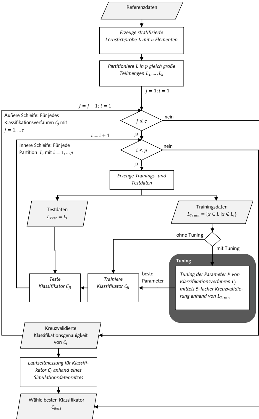
Abb. 7-14: Ablaufdiagramm der Modellselektion
