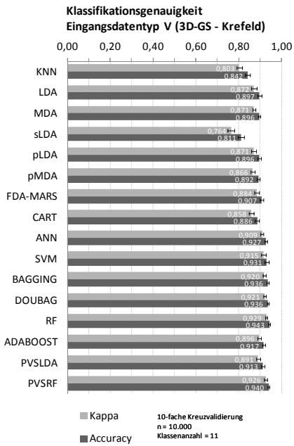
Abb. D-2: Klassifikationsgenauigkeit (Overall Accuracy und Kappa) für den Eingangsdatentyp V
