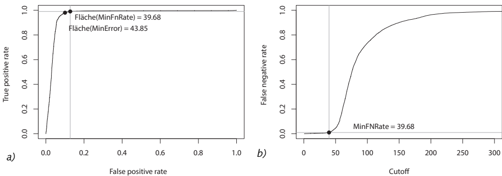
Abb. 8-7: Ermittlung des optimierten Schwellwertes angebaute Nebengebäude: a) ROC-Kurve (links) mit optimalen Schwellwert für Methode 1 (MinFnRate) und Methode 2 (MinError) und b) Kurve der Fehlerrate für Methode 2
