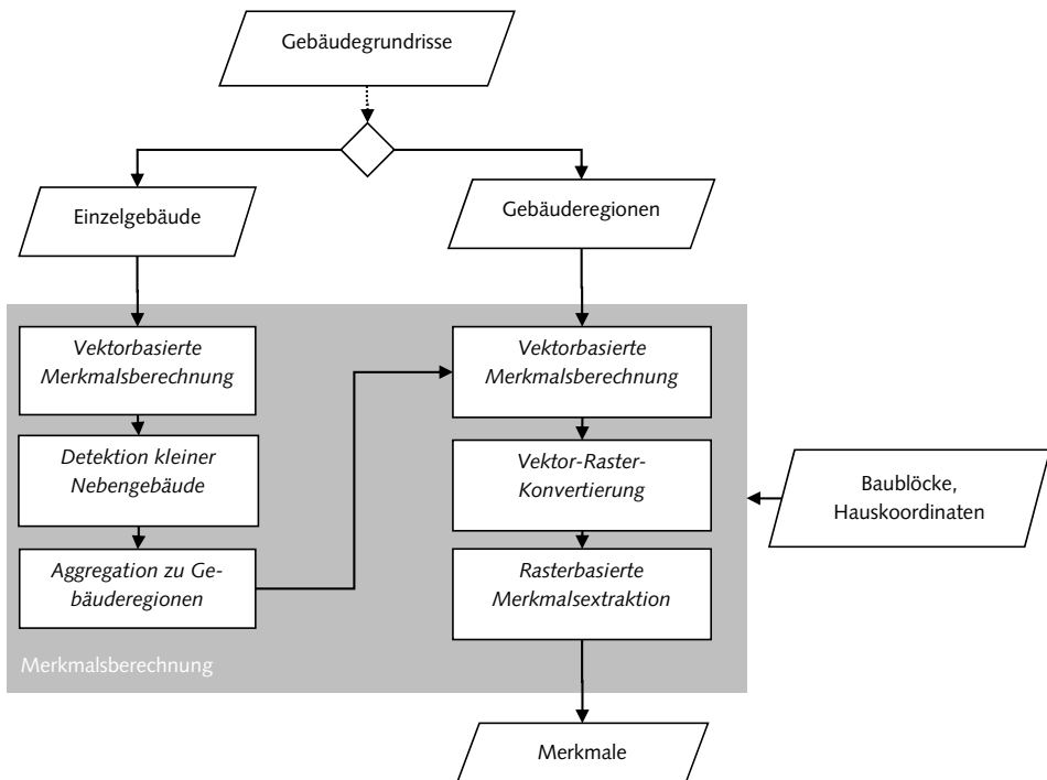
Abb. 7-10: Workflow der Merkmalsberechnung
