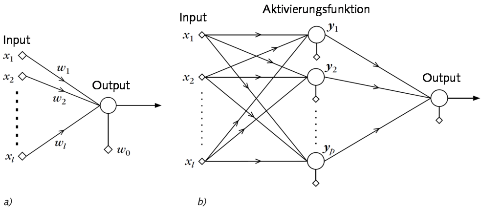
Abb. 3-8: Einlagiges Netz als einfaches lineares Regressionsmodell (links) und das Standardnetzwerk mit drei Schichten (Abgeänderte Graphik nach Theodoridis & Koutroumbas, 2008)
