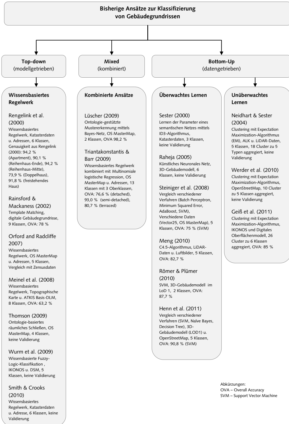
Abb. 4-1: Überblick über die Ansätze zur Klassifizierung individueller Gebäudegrundrisse
