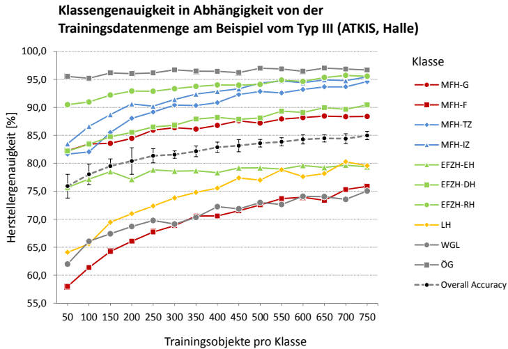
Abb. 8-17: Klassengenauigkeit in Abhängigkeit von der Anzahl an Trainingsbeispielen pro Klasse. Die Herstellergenauigkeit wurde durch 10-fach wiederholtes Trainieren und Testen ermittelt.
