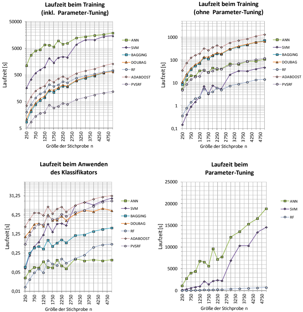
Abb. 8-12: Ergebnisse der Laufzeitmessung ausgewählter Methoden (logarithmisch skalierte Vertikalachse)
