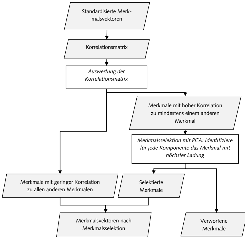
Abb. 7-12: Workflow der Merkmalsselektion
