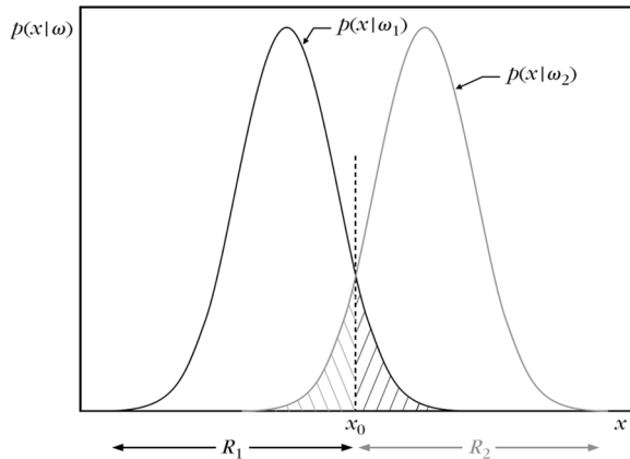
Abb. 3-5: Eindimensionale Verteilungsdichten zweier normalverteilter Klassen mit gleicher Varianz und Aufteilung des Merkmalsraums in zwei Regionen R_1 und R_2 (Quelle: Theodoridis & Koutroumbas, 2008)
