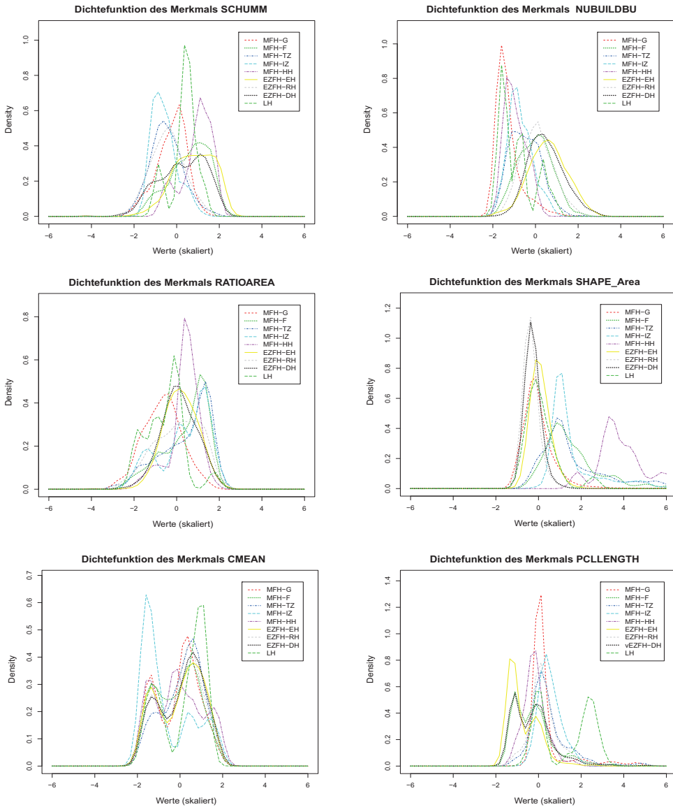
Abb. 8-8: Wahrscheinlichkeitsdichtefunktionen der Wohngebäudeklassen am Beispiel ausgewählter Merkmale. Datengrundlage sind die standardisierten Merkmalsvektoren des Datensatzes von Krefeld (ALK).
