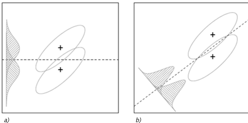
Abb. 3-7: Beste Hyperebene der LDA: a) Maximierung des Abstandes der Mittelpunkte und b) optimale Projektionsrichtung nach Fisher-Kriterium (Quelle: Hastie et al., 2009)
