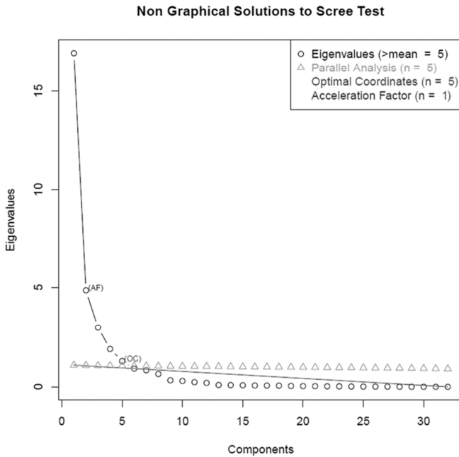
Abb. 7-13: Scree-Plot und Anzahl der extrahierten Komponenten mittels verschiedener Kriterien (Quelle: Eigene Darstellung unter Nutzung des R Packages „nFactors“)
