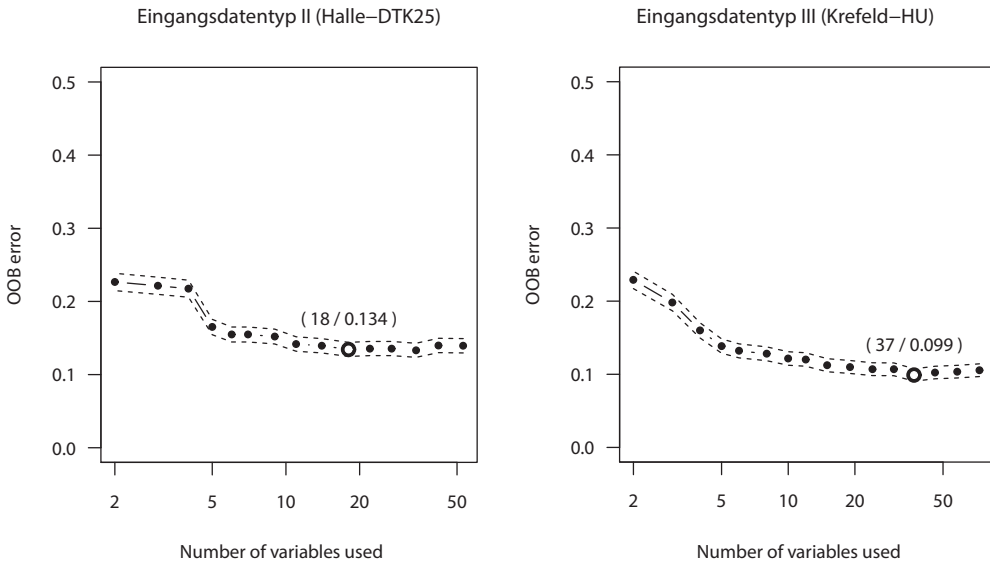
Abb. 8-20: OOB-Fehler in Abhängigkeit der Merkmalsanzahl am Beispiel der Eingangsdatentypen II (links) und III (rechts). Die beste Merkmalsmenge ist hervorgehoben.
