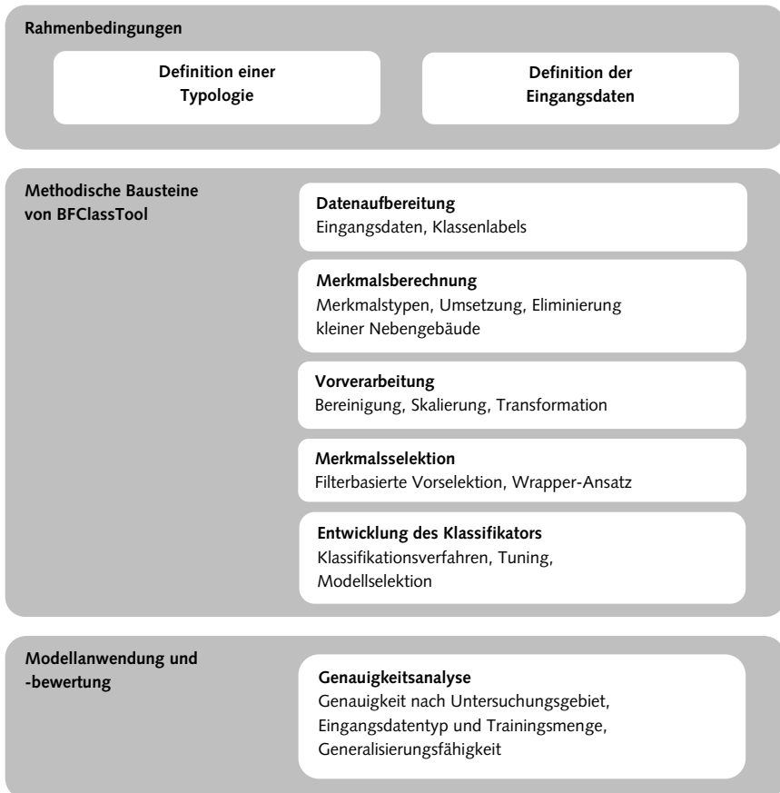
Abb. 7-1: Design der Verfahrensentwicklung
