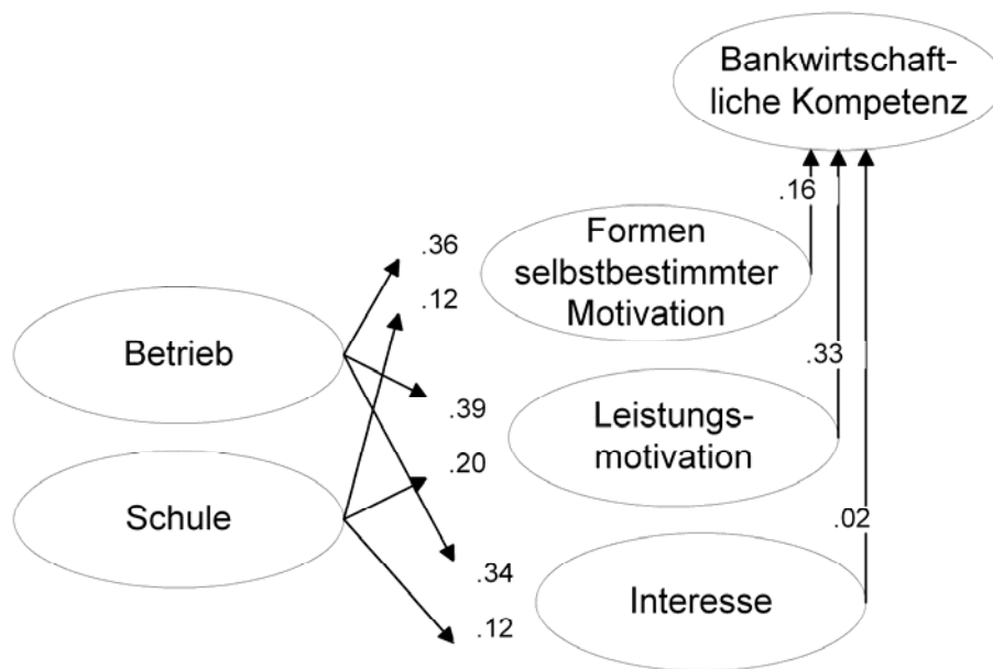
Abbildung 3: LISREL-Modell Umgebungsbedingungen, motivationale Orientierungen und bankwirtschaftliche Kompetenz
