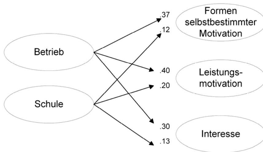
Abbildung 1: Partialkorrelationen Ausbildungsbedingungen – motivationale Orientierungen
