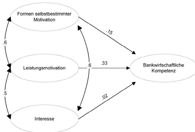
Abbildung 2: Partialkorrelationen motivationale Orientierungen – bankwirtschaftliche Kompetenz
