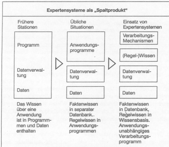
Abb. 5: Evolution von Softwarearchitekturen (Quelle: Maciejewski, P.G., 1989: Künstliche Intelligenz. Heidelberg, S. 32).
