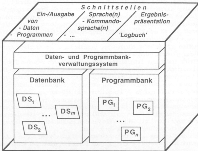
Abb. 1: Architektur eines statistischen Daten- und Programmbanksystems (DS: Datenstruktur; PG: Programmgruppe). (Quelle: Haag, U./Haux, R./Kieser, M., 1992: Statistische Auswertungssysteme. Stuttgart/Jena/New York: G. Fischer, S. 13).
