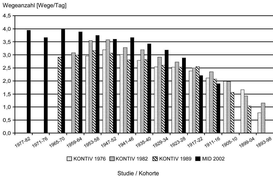
Abb. 5: Wegezahlnachtag nach Geburtskohorten
