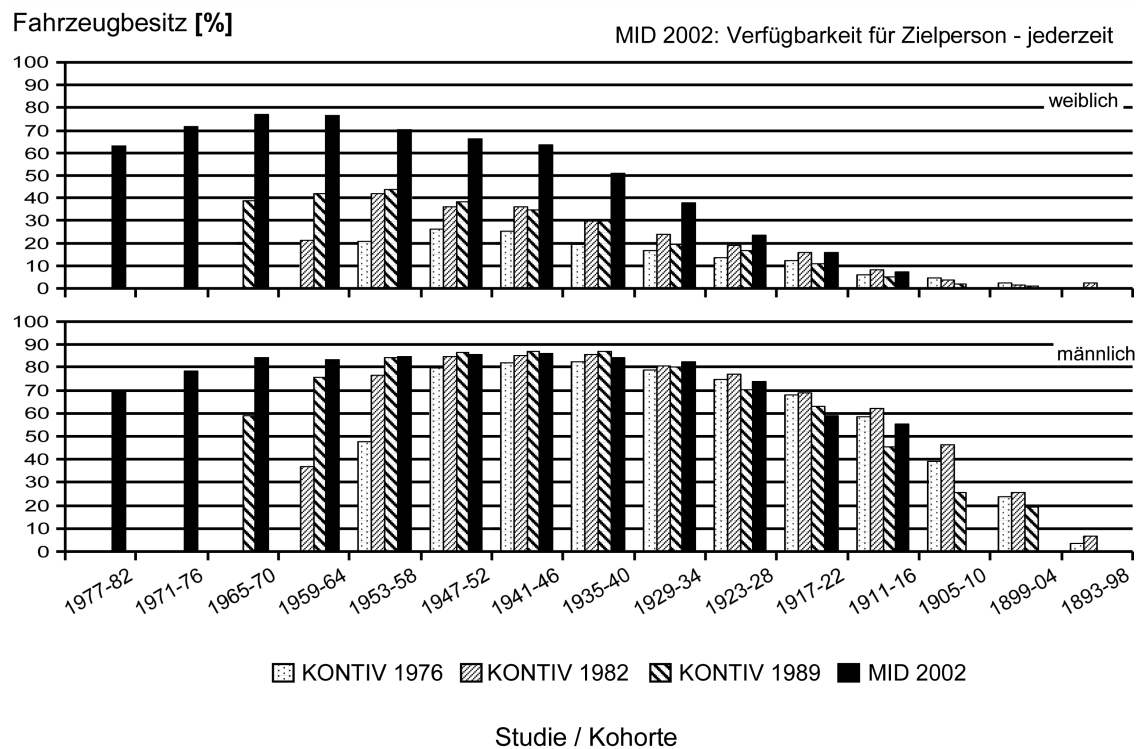
Abb. 4: Fahrzeugbesitz/-verfügbarkeit nach Geburtskohorten und Geschlecht
