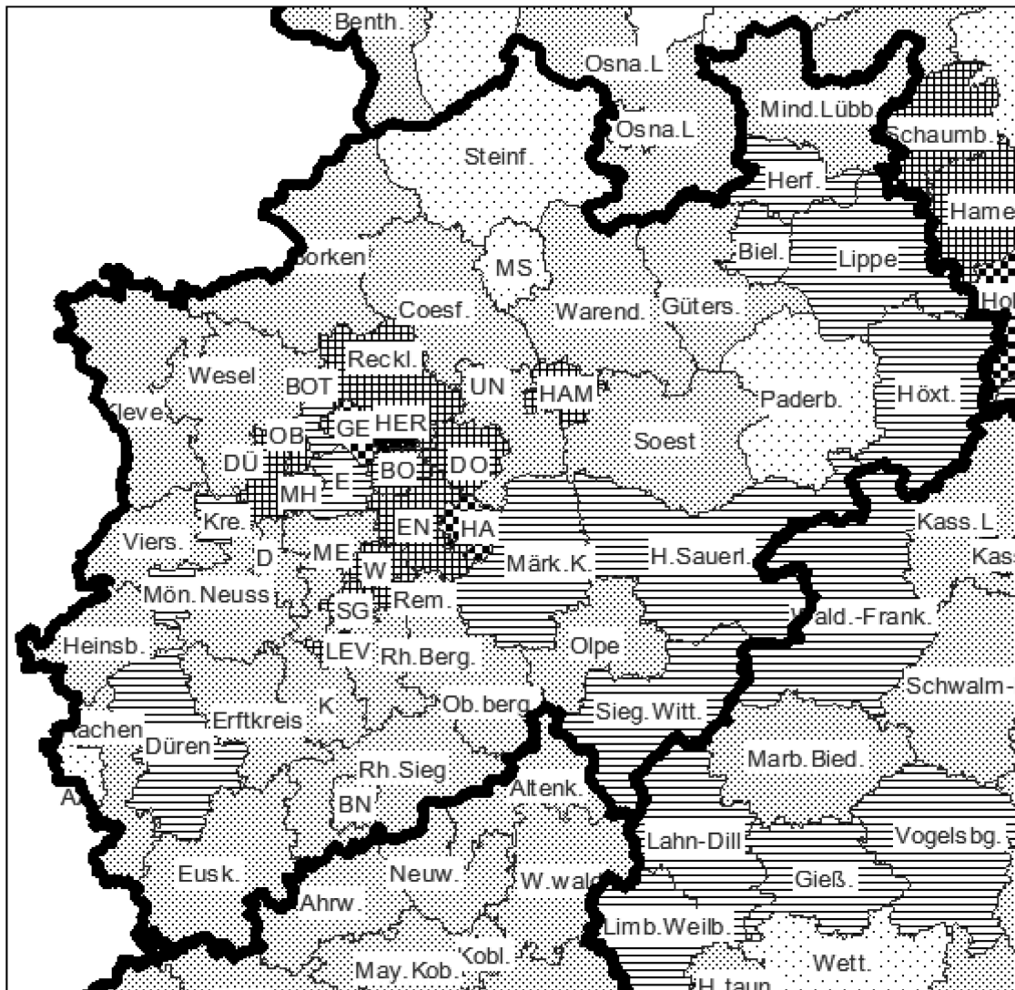
Abb. 3: Prognose der Erwerbstätigkeit in den Kreisen und kreisfreien Städten 2001–2010
