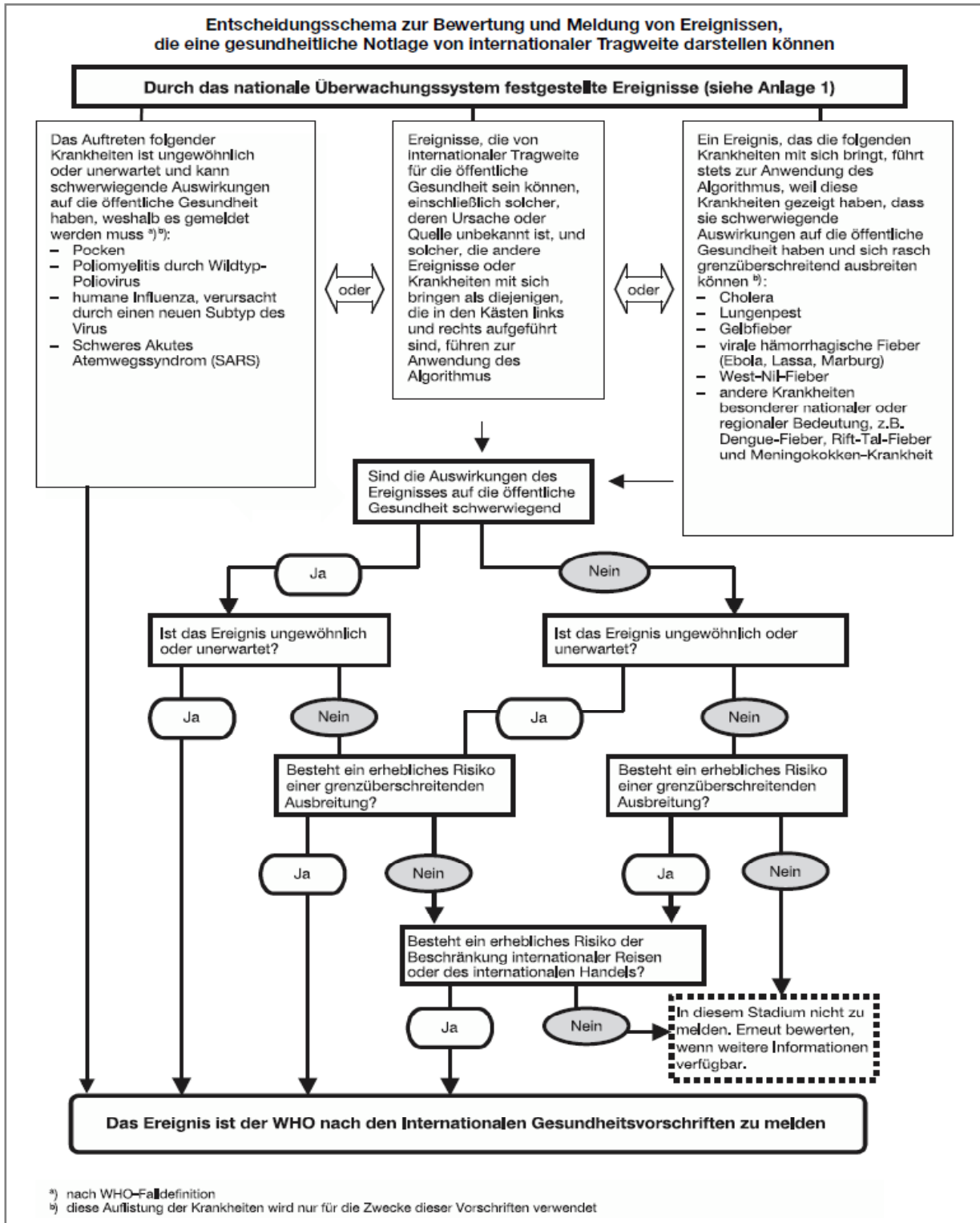
Schaubild 1: Entscheidungsinstrument
