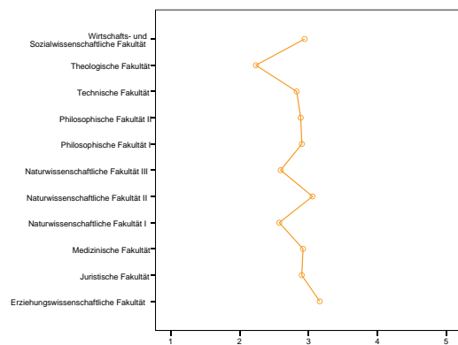
Abbildung 5.4: motivierend–demotivierend
