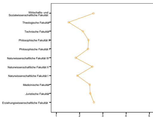
Abbildung 5.1: positiv–negativ
