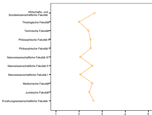
Abbildung 5.3: angenehm–unangenehm
