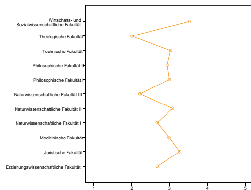
Abbildung 5.2: persönlich–unpersönlich
