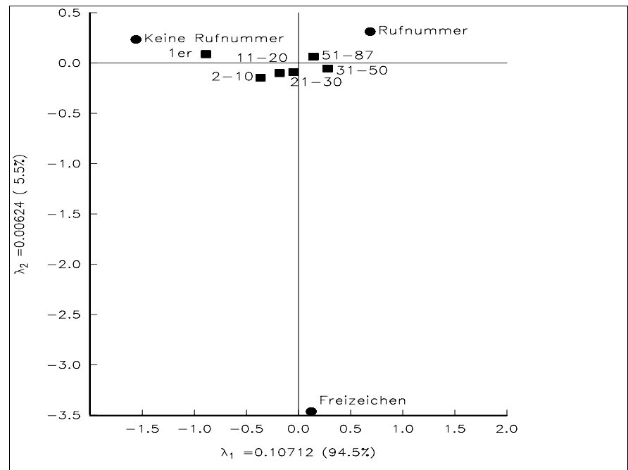
Abbildung 2: Korrespondenz zwischen Blockbesetzung und den Stati der Ziffernfolgen
