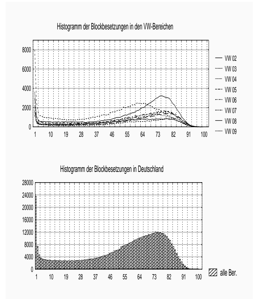
Abbildung 1: Blockbesetzungen in den Vorwahlbereichen und in Deutschland insgesamt
