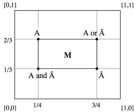
Fig. 1.1. Fuzzy cube
