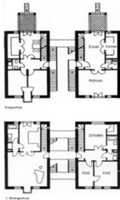
Abbildung 7: Haus 9, Brandt, Heiß, Liepe, Steigelmann, EG + OG
