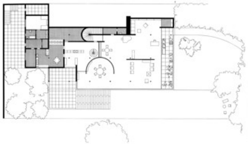
Abbildung 4: Haus Tugendhat, Grundriss EG
