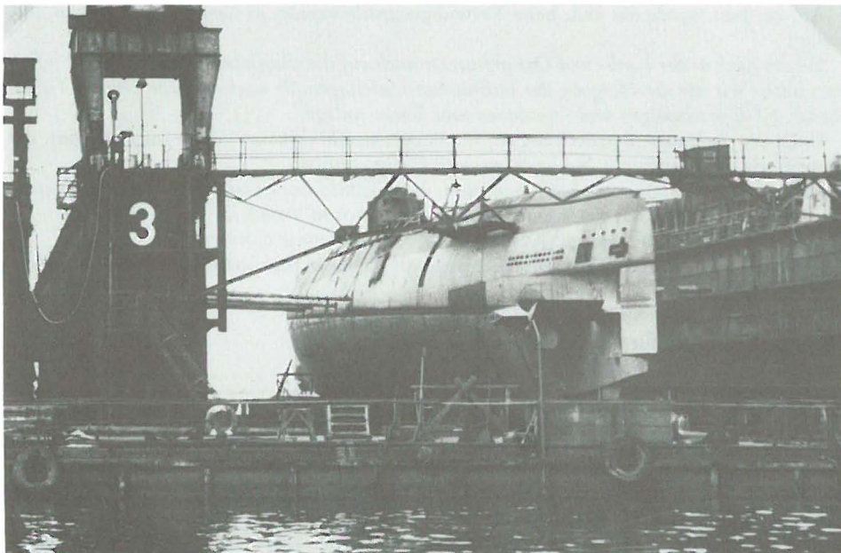
U WAL (U 2540) nach dem ersten Bauabschnitt im September 1959 bei der Dockbesichtigung im Schwimmdock 3 der Kieler Howaldtswerke
