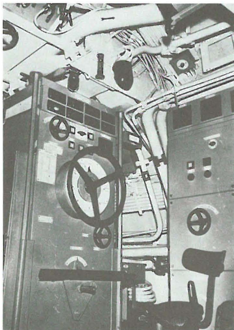
Fahrstand der Bb. E Maschine, daneben die Generator Schalttafel. (Foto HDW)
