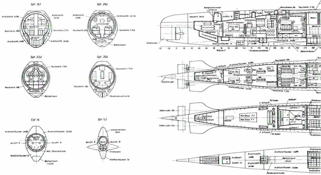
Quer- und Längsschnitte durch U-WILHELM BAUER. (Ausführung 1962)
