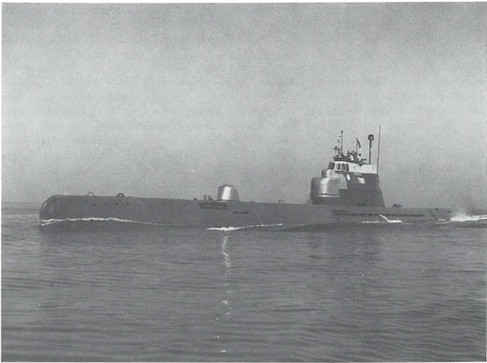
U-WILHELM BAUER im Jahre 1976 mit ausgefahrener Radarantenne und zusätzlicher kipbarer Stabantenne an Bb. (Foto Conen)
