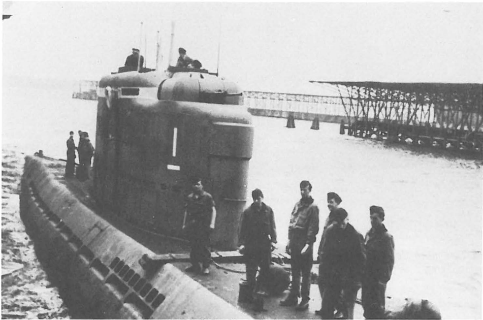
Ein Blohm & Voss-U Boot des Typs XXI bei der UAK Erprobung in Kiel
