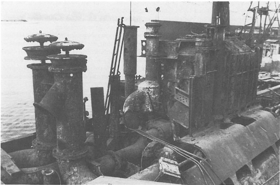
Turm von U 2540 nach Abnahme der Verkleidung Anfang 1958. Im Vordergrund Dieselluftmaste, Stabantennenrohr, Abluftmast und die Führungsrohre für den Schnorchelmast. (Foto HDW)
