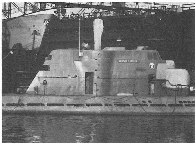
WILHELM BAUER nach Überholung und Umbau im Oktober 1969 mit einem neuen Schnorchel bei HDW in Kiel Gaarden. (Foto Nöcker)
