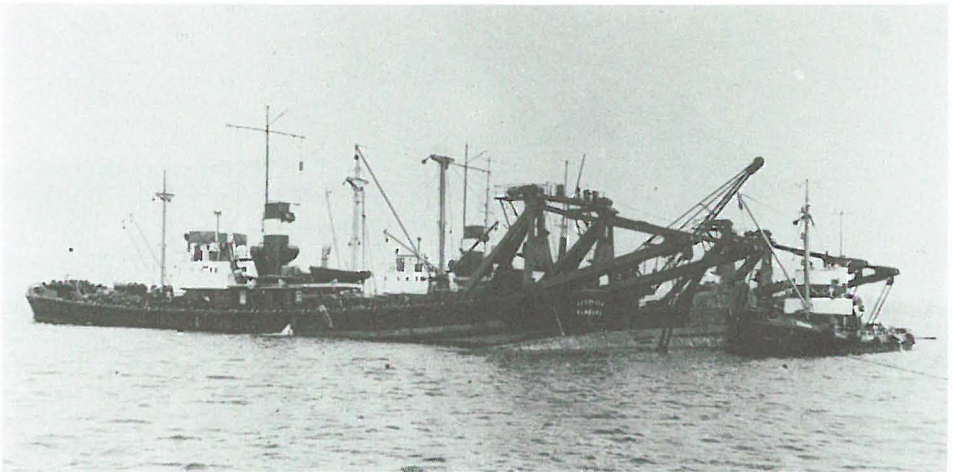
U 2540 nach der Hebung im Juni 1957 an den Trossen der Bergungsschiffe ENERGIE und AUSDAUER
