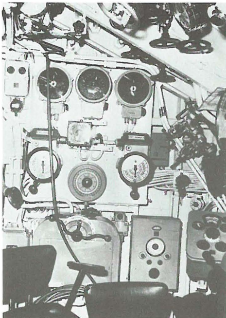
Seitenruderstand in der Zentrale (Foto HDW)
