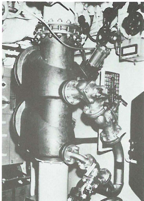
Durchführung des Schnorchelmastes in der Zentrale. (Foto HDW)
