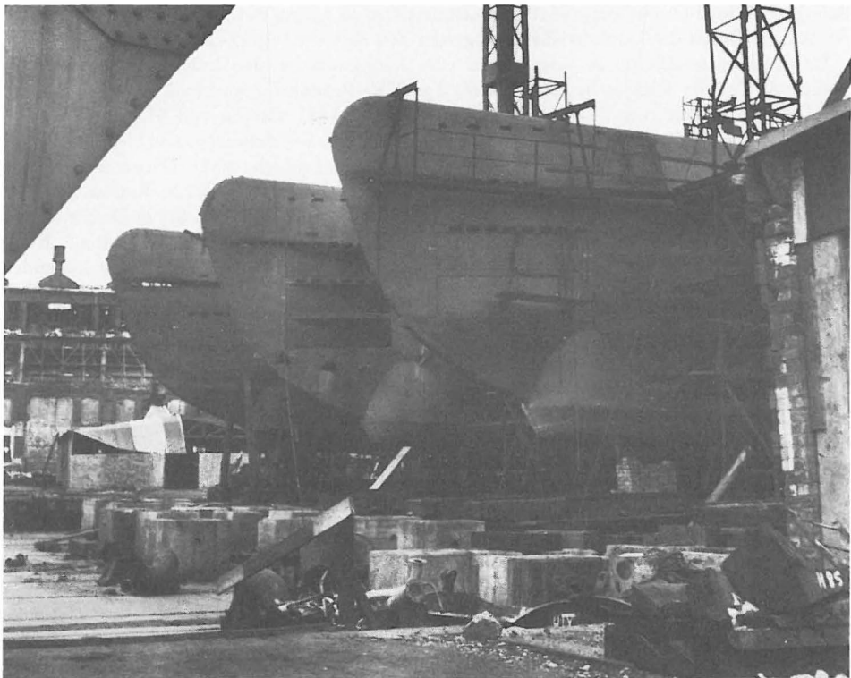
Der Bauplatz von U 2540 bei Blohm & Voss. Zu erkennen sind die Bugteile von U 2564, 2562 und 2560 auf Helling 9. Vor U 2560 war hier U 2540 zusammengebaut worden.
