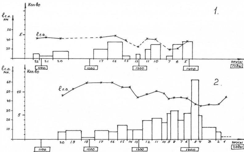
Abb. 6 Stratigraphische Verteilung der Beschlagklammern vom Typ 1: Arithmetischer Mittelwert für die Rückenlänge (l.c.a.). 1: Ausgrabung von Michailowsk; 2: Ausgrabung von Nutnyi.
