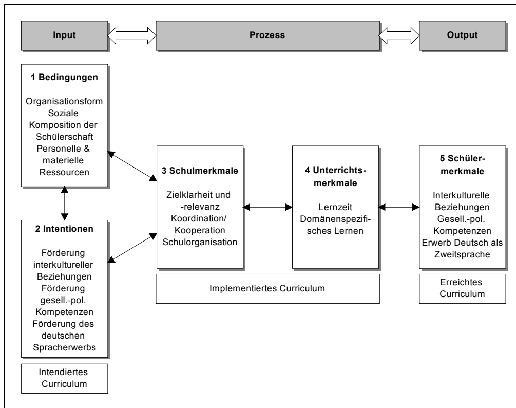
Abb. 1: Untersuchungsleitendes Modell
