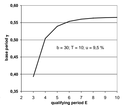
Figure 8c : (E, \gamma)
