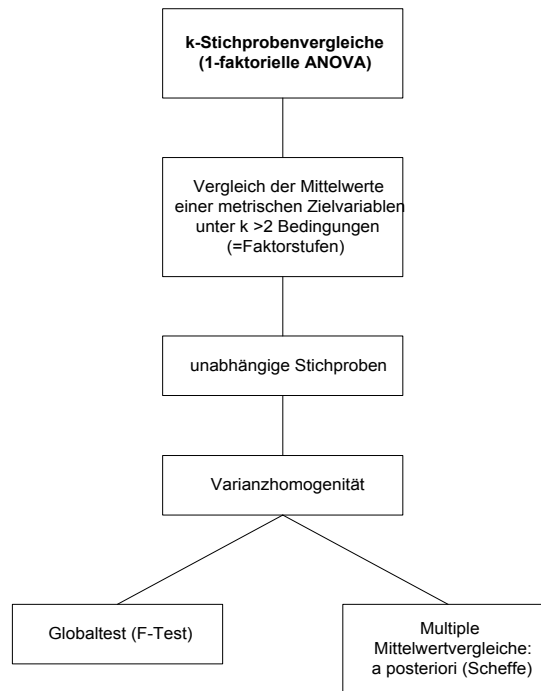
Abbildung 13: Ablauflogik einer einfaktoriellem Varianzanalyse
