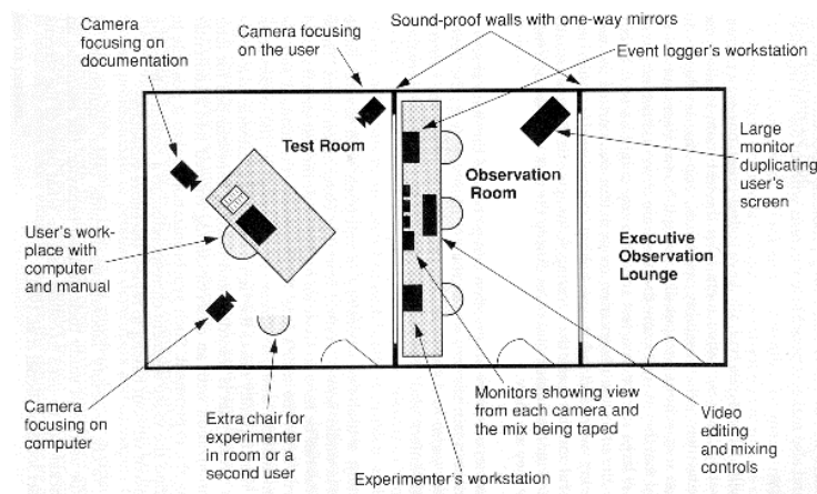
Abbildung 4: Usability-Labor (Nielsen 1993:201)
